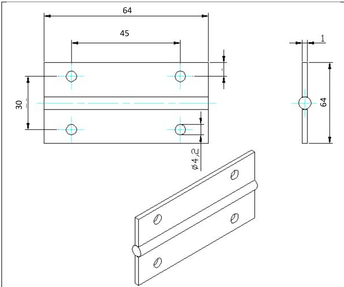
ΣΤΟΙΧΕΙΟ ΣΥΝΔΕΣΗΣ (ΣΥΝΔΕΣΜΟΣ)
