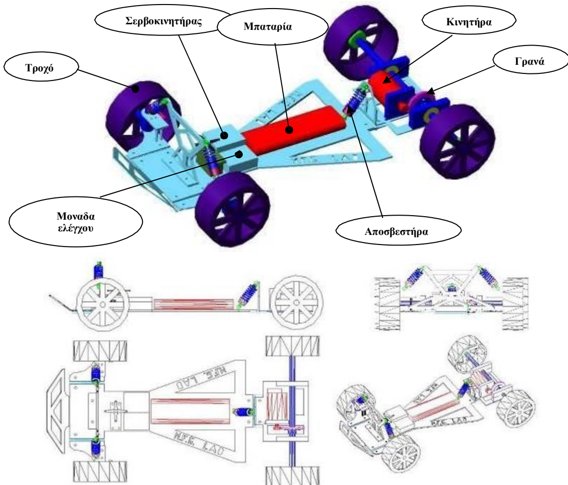
Σχήμα 3: Τηλεκατευθυνόμενο όχημα
