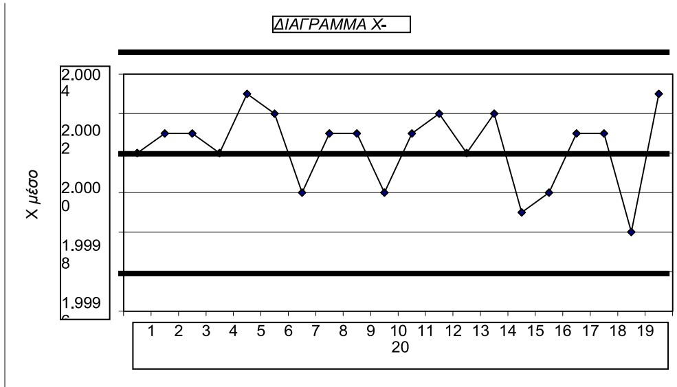
Σχήμα 2.7: Διάγραμμα \bar{X}
