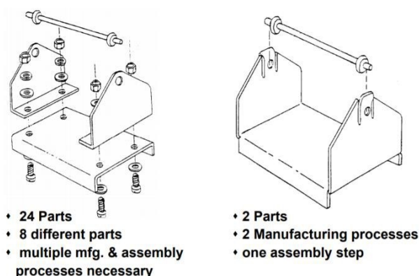
Σχήμα 5.4: Μείωση αριθμού εξαρτημάτων
