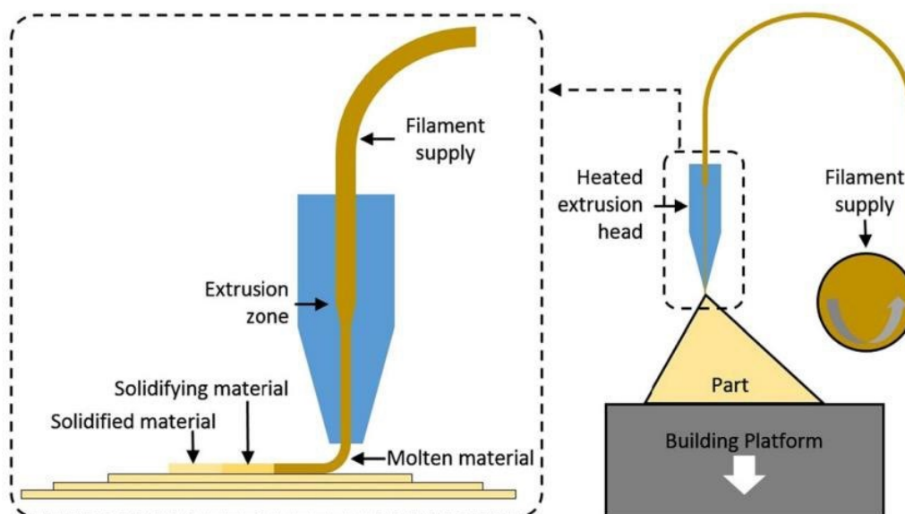
Σχήμα 4.9: Κατασκευή με εναπόθεση ημίρρευστου υλικού
