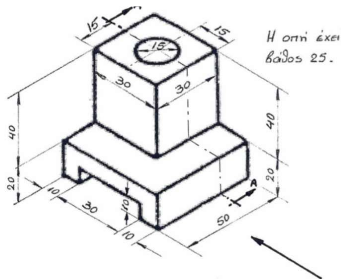
Σχέδιο 7. Βάση μηχανής.
