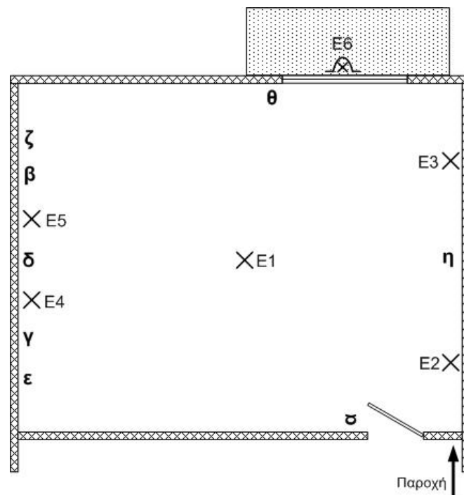
Σχήμα 1: Κάτοψη τμήματος οικίας
