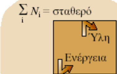
E = \text{σταθερό} Απομονωμένο (γ)
