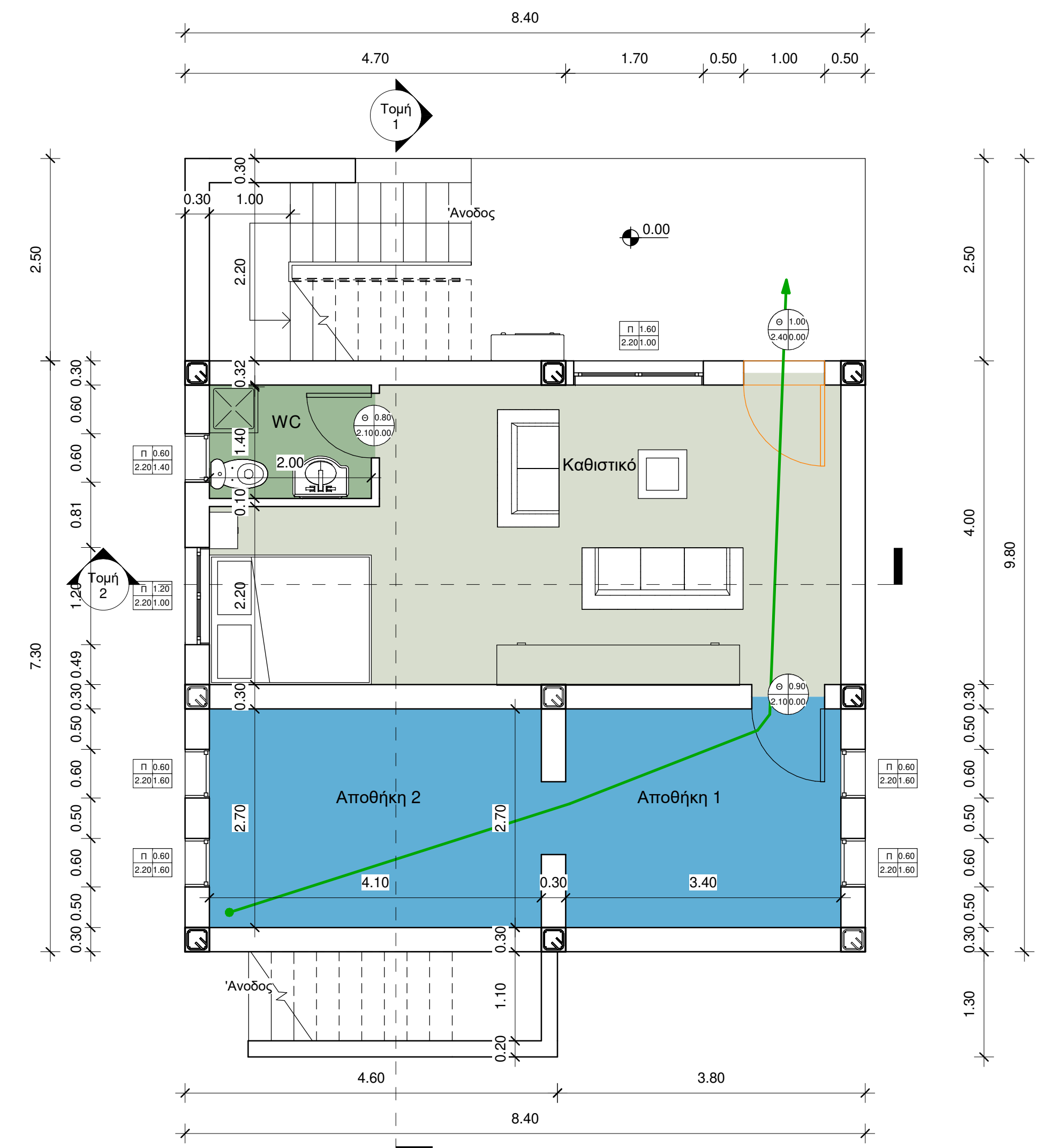
02 2 - Οδευση διαφυγής 1 : 50
