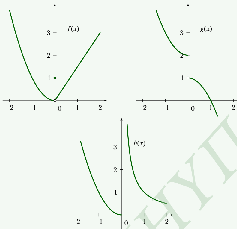
Σχήμα 8.5: Είδη ασυνέχειας
