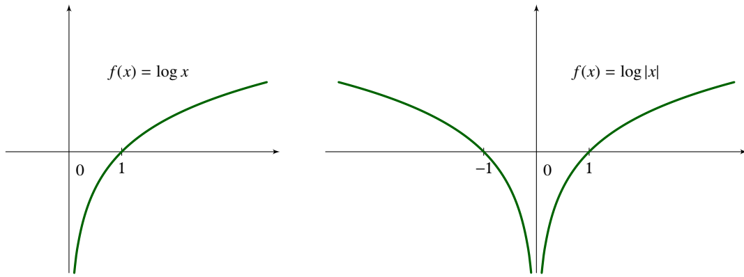
Σχήμα 7.40: Η λογαριθμική συνάρτηση f(x) = \log x και η f(x) = \log |x|
