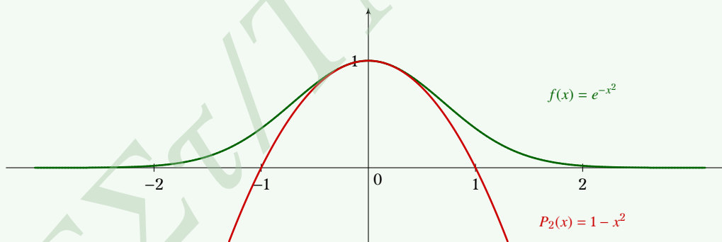
Σχήμα 9.5: e^{-x^2} \approx 1 - x^2 γύρω από το x = 0
