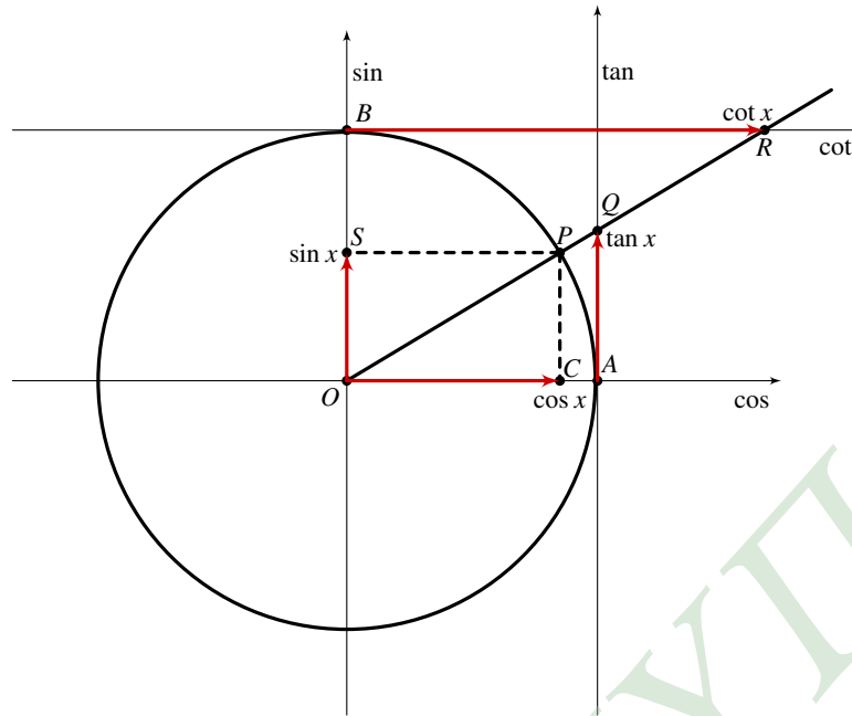
Σχήμα 7.9: Ο τριγωνομετρικός κύκλος II
