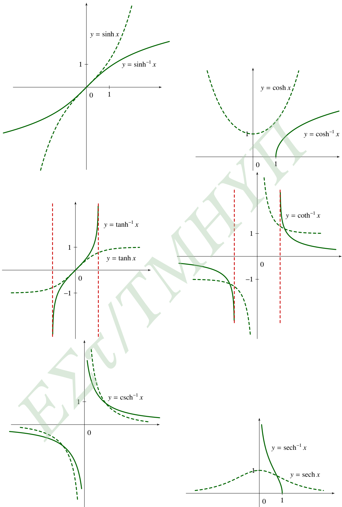
Σχήμα 7.44: Οι αντίστροφες υπερβολικές συναρτήσεις \sinh^{-1} x , \cosh^{-1} x , \tanh^{-1} x , \coth^{-1} x , \operatorname{csch}^{-1} x και \operatorname{sech}^{-1} x
