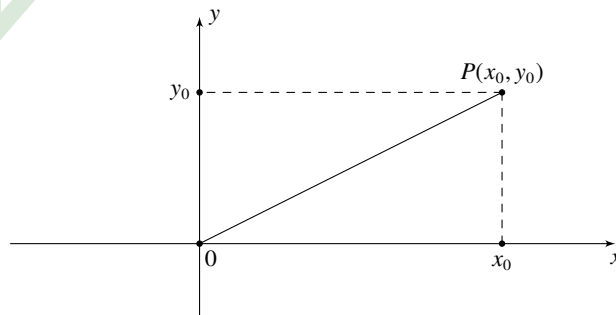
Σχήμα 4.1: Το καρτεσιανό επίπεδο.
