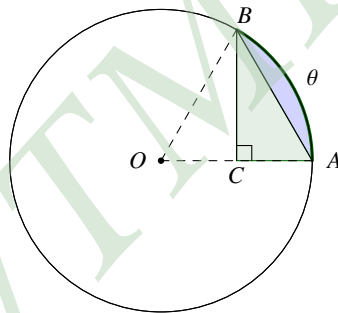
Σχήμα 9.18: Άσκηση 28
