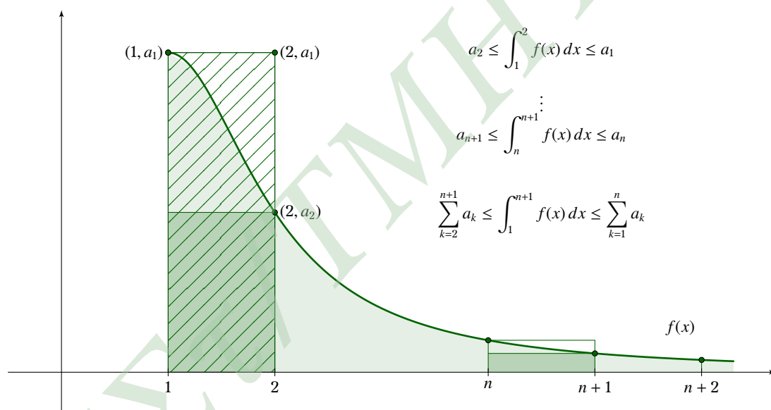
Σχήμα 10.7: Το κριτήριο του ολοκληρώματος
