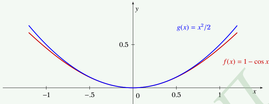
Σχήμα 9.4: Για μικρές τιμές του |x| είναι 1 - \cos x \approx x^2/2
