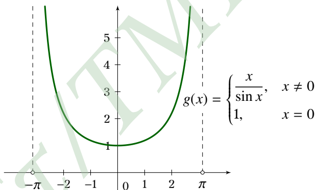
Σχήμα 9.14: Η συνάρτηση g στο (-\pi, \pi)
