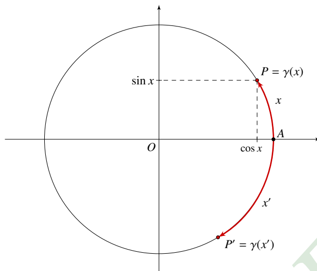
Σχήμα 10.6: Τόξο και μήκος τόξου
