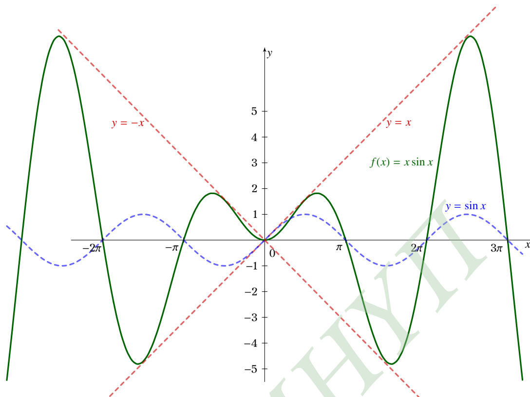
Σχήμα 7.29: Η συνάρτηση f(x) = x \sin x
