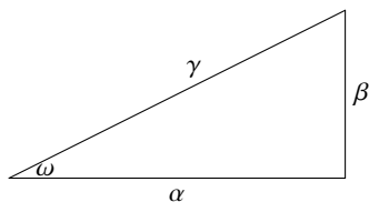
Σχήμα 7.2: Τριγωνομετρικοί αριθμοί γωνίας
