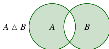
Σχήμα 1.3: Η συμμετρική διαφορά A \Delta B δύο συνόλων A και B .
