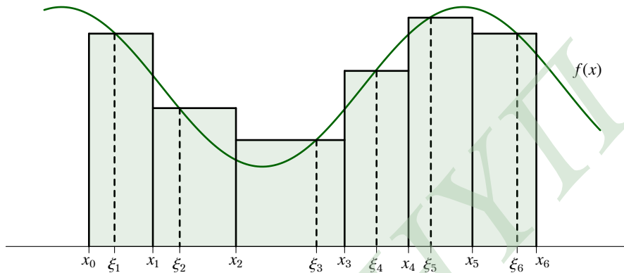
Σχήμα 10.1: Το άθροισμα Riemann ( N = 6 , a = x_0 , b = x_6 )
