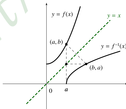
Σχήμα 7.13: Οι συναρτήσεις y = f(x) και y = f^{-1}(x)
