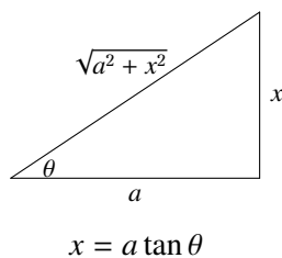
Σχήμα 10.4: Τριγωνομετρικές αντικαταστάσεις
