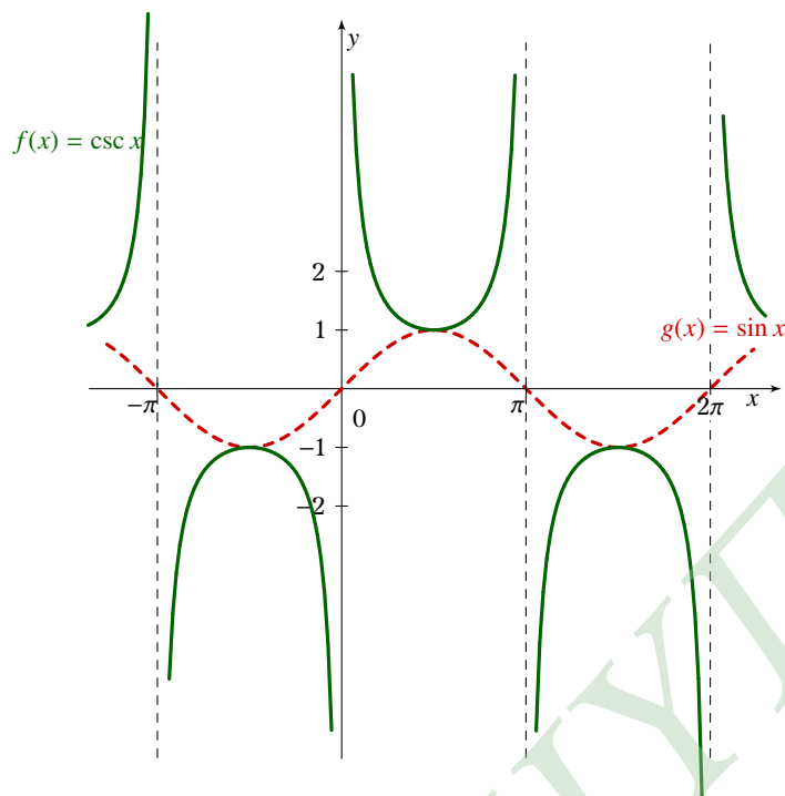
Σχήμα 7.32: Η συνάρτηση f(x) = \csc x
