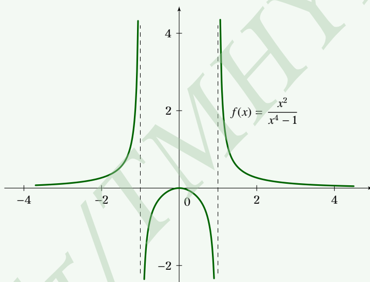
Σχήμα 7.25: Η συνάρτηση f(x) = x^2/(x^4 - 1)
