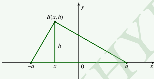
Σχήμα 9.8:
