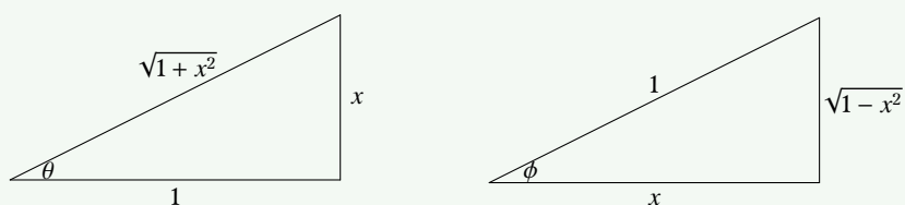
Σχήμα 7.37: Βοηθητικά τρίγωνα
