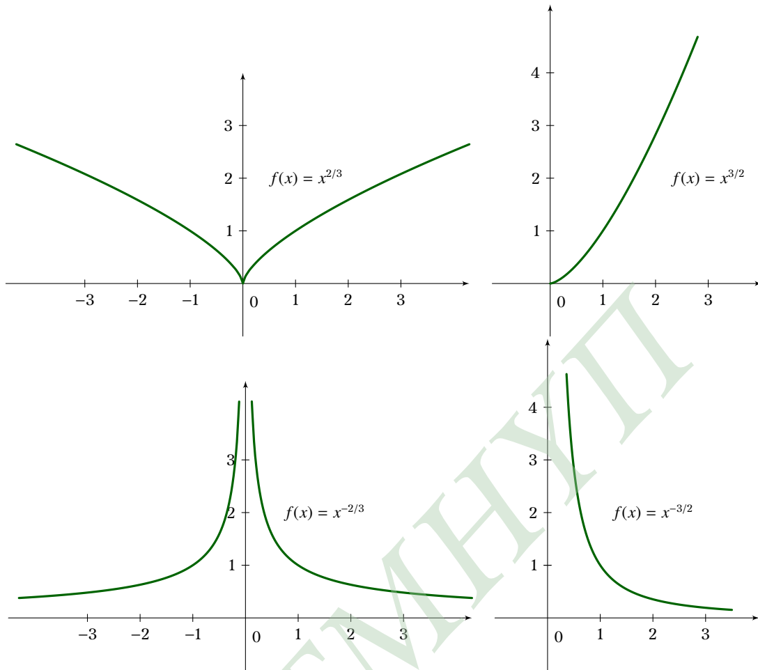
Σχήμα 7.19: Οι συναρτήσεις f(x) = x^{2/3} , f(x) = x^{3/2} , f(x) = x^{-2/3} και f(x) = x^{-3/2}
