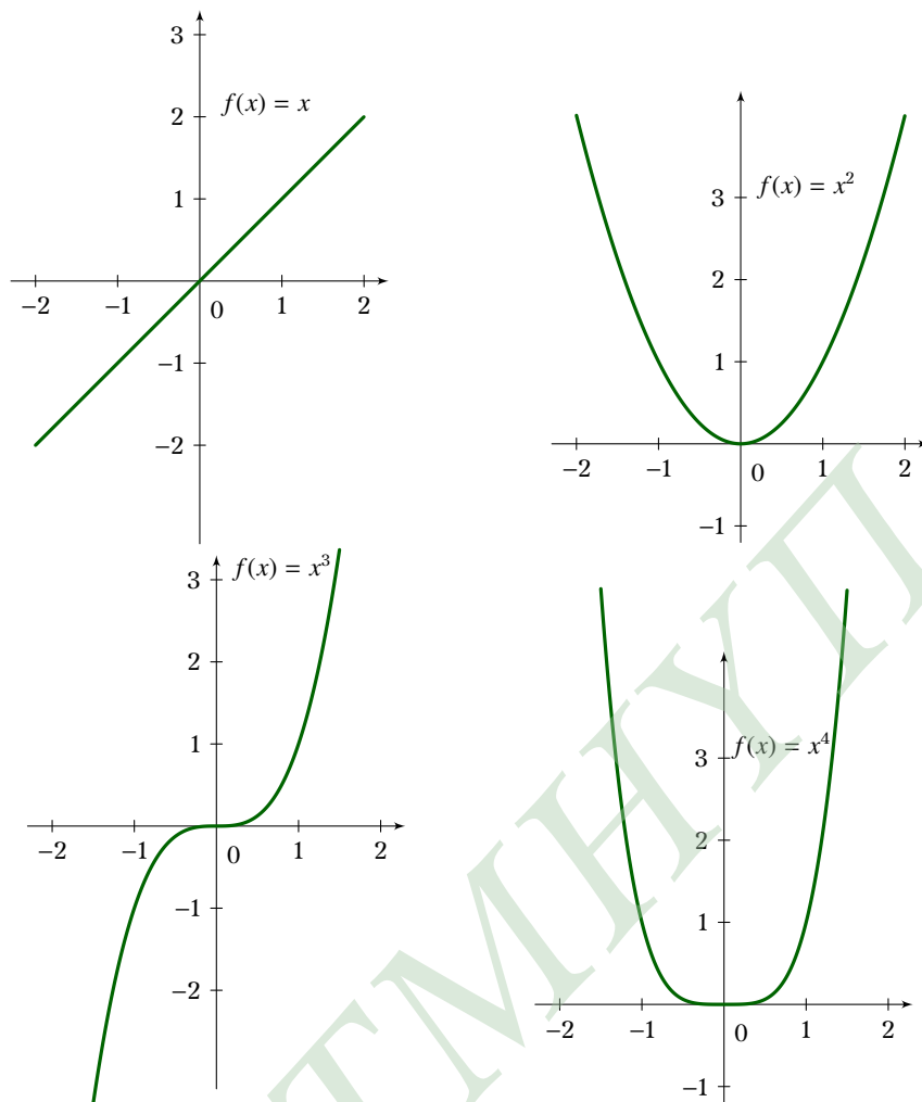
Σχήμα 7.16: Οι συναρτήσεις f(x) = x^n , για n = 1, 2, 3, 4
