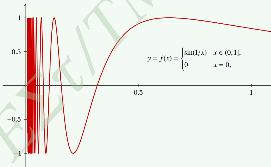
Σχήμα 9.13: Μια μη συνεχής συνάρτηση η οποία έχει την ιδιότητα Darboux
