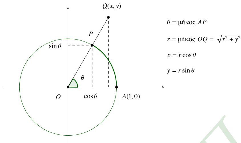
Σχήμα 7.10: Καρτεσιανές και πολικές συντεταγμένες
