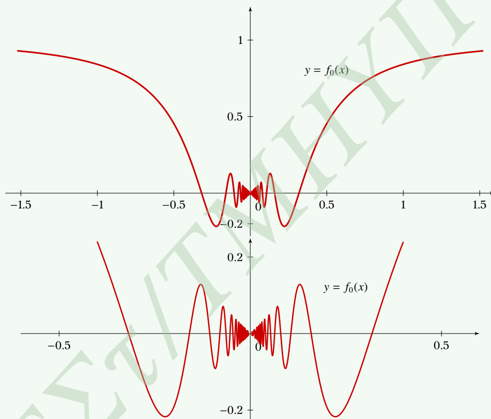
Σχήμα 8.2: Η συνάρτηση f_0(x) = x \sin(1/x) , x \neq 0 και f_0(0) = 0
