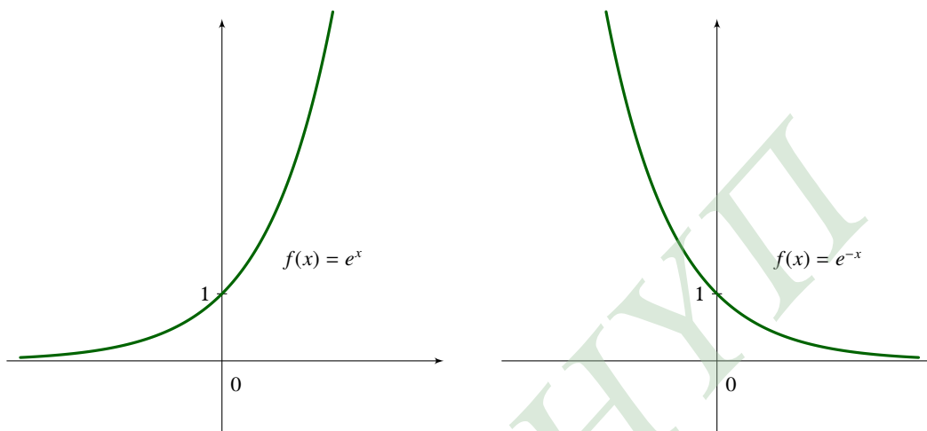
Σχήμα 7.39: Οι εκθετικές συναρτήσεις f(x) = \exp x και f(x) = (1/e)^x = e^{-x} = \exp(-x)
