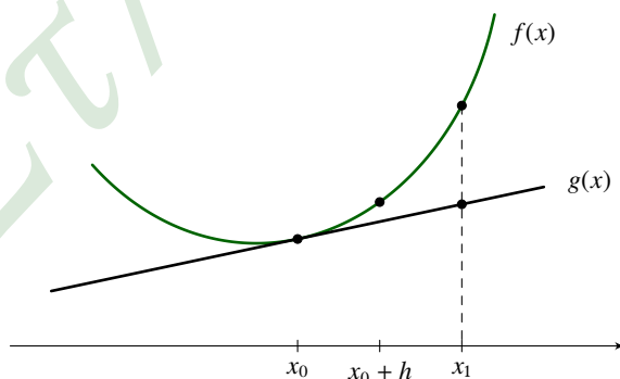
Σχήμα 9.11: Η εφαπτόμενη ευθεία στη γραφική παράσταση κυρτής συνάρτησης
