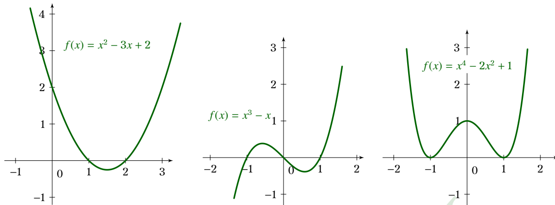
Σχήμα 7.21: Χαρακτηριστικές πολυωνυμικές συναρτήσεις
