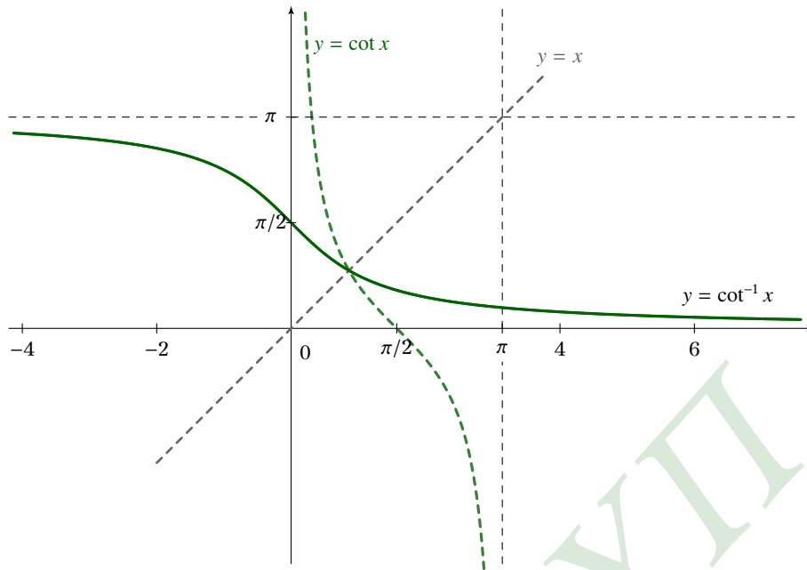
Σχήμα 7.36: Η συνάρτηση \cot^{-1}
