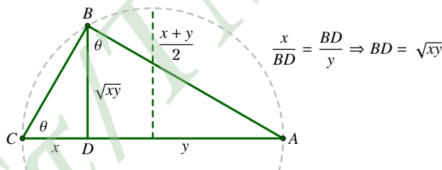
Σχήμα 7.42: \sqrt{xy} \leq (x+y)/2 .
