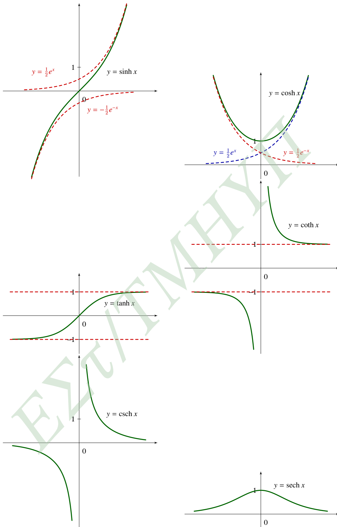
Σχήμα 7.43: Οι υπερβολικές συναρτήσεις \sinh x , \cosh x , \tanh x , \coth x , \operatorname{csch} x και \operatorname{sech} x
