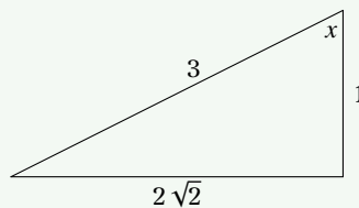
Σχήμα 7.34:
