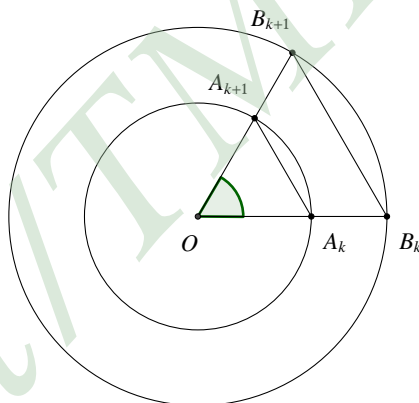
Σχήμα 7.5: Ομοιότητα τριγώνων
