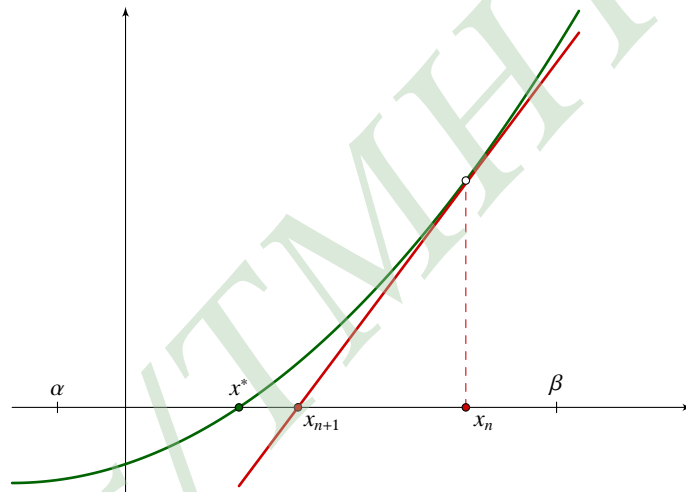
Σχήμα 9.7: Γεωμετρική αναπαράσταση για το σχήμα του Newton
