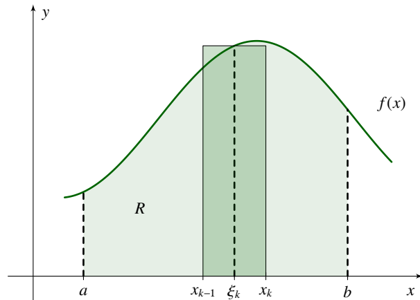
Σχήμα 10.5: Το σκιασμένο ορθογώνιο με βάση [x_{k-1}, x_k] και ύψος f(\xi_k)
