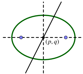
Σχήμα 9.3: Άσκηση 9.8
