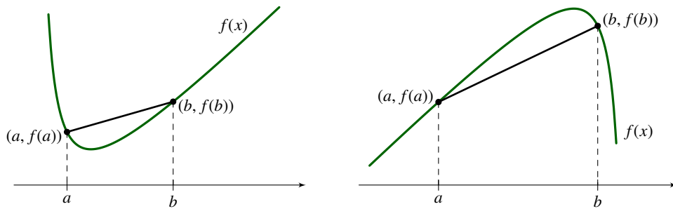
Σχήμα 9.9: Μια κυρτή συνάρτηση f , και μια κοίλη συνάρτηση f
