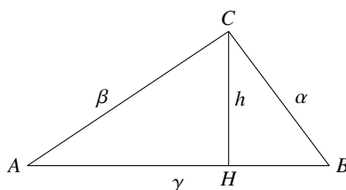
Σχήμα 7.3: Ο νόμος των ημιτόνων
