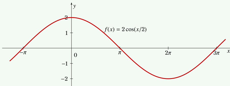
Σχήμα 7.28: Η συνάρτηση f(x) = 2 \cos(x/2)
