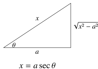
Σχήμα 10.4: Τριγωνομετρικές αντικαταστάσεις
