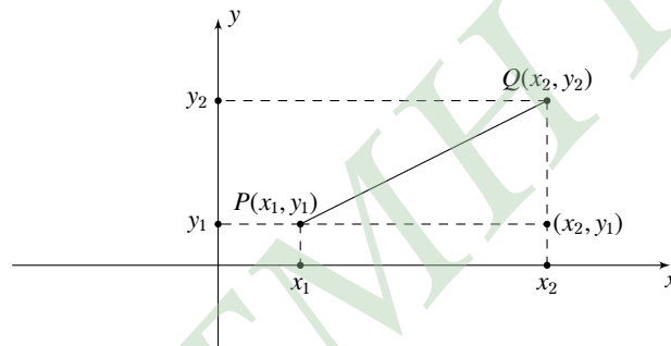
Σχήμα 7.1: Απόσταση στο επίπεδο
