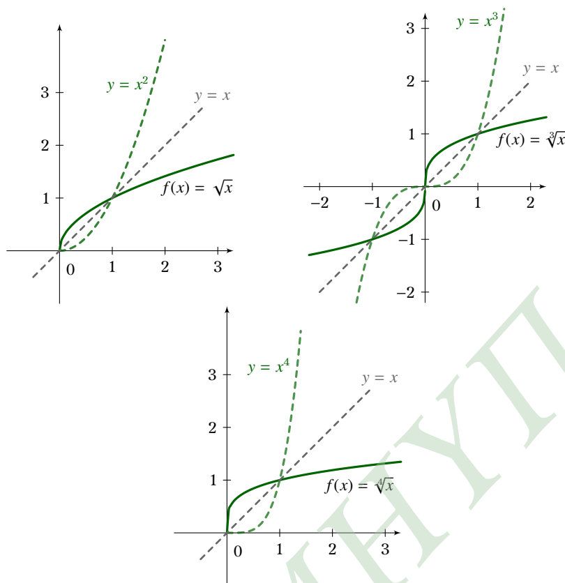
Σχήμα 7.18: Οι συναρτήσεις f(x) = \sqrt{x} , f(x) = \sqrt[3]{x} και f(x) = \sqrt[4]{x}
