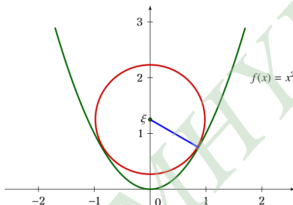
Σχήμα 9.15: Άσκηση 10
