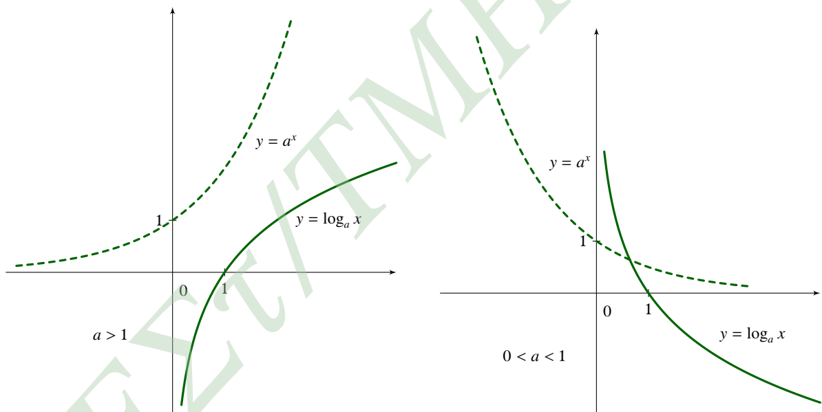
Σχήμα 7.41: Η λογαριθμική συνάρτηση f(x) = \log_a x
