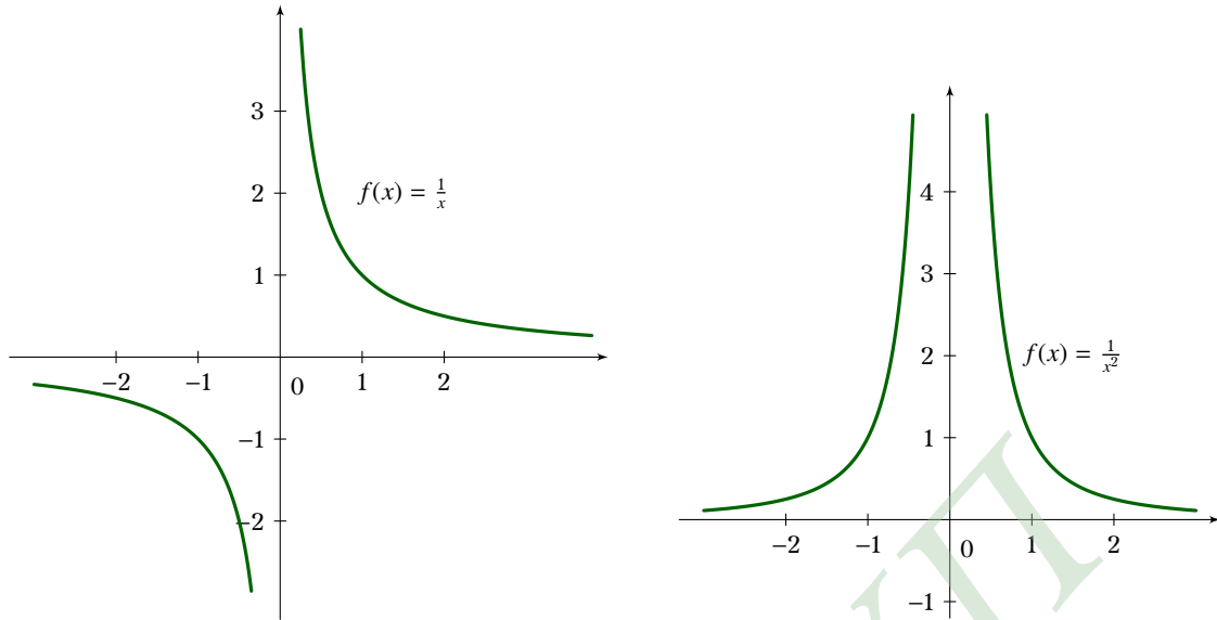
Σχήμα 7.17: Η συναρτήσεις f(x) = x^{-n} για n = 1, 2
