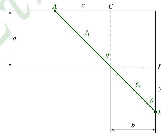
Σχήμα 9.16: Άσκηση 18
