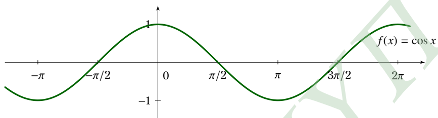
Σχήμα 7.26: Η συνάρτηση f(x) = \cos x
