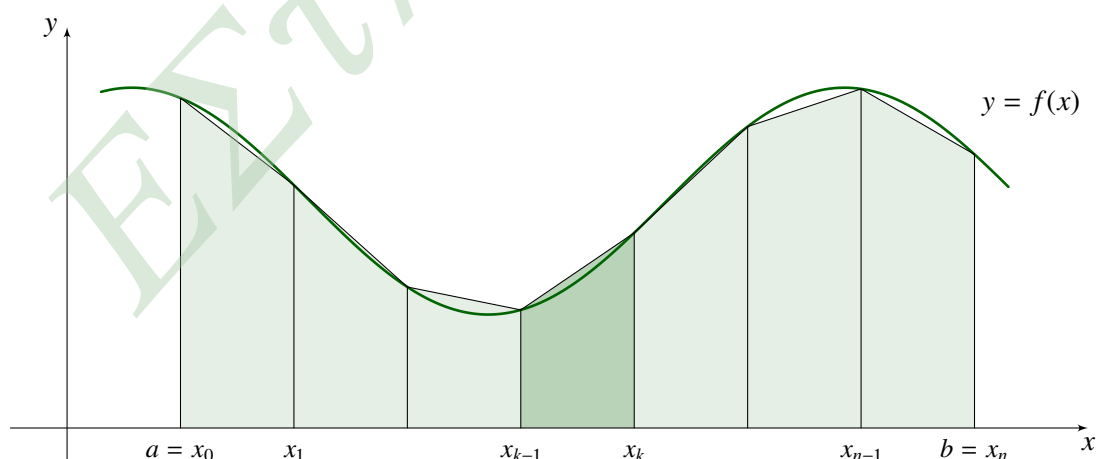
Σχήμα 10.2: Ο κανόνας του τραπεζίου
