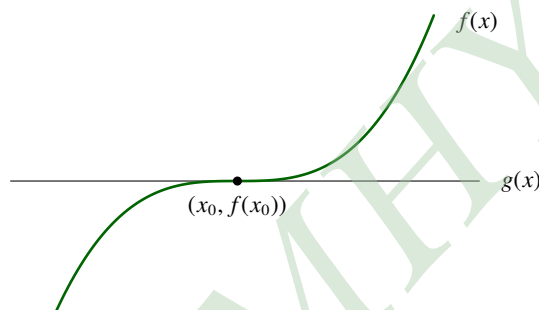
Σχήμα 9.12: Η εφαπτόμενη ευθεία στη γραφική παράσταση συνάρτησης σε σημείο καμπής
