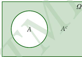
Σχήμα 1.2: Το συμπλήρωμα A^c του συνόλου A .
