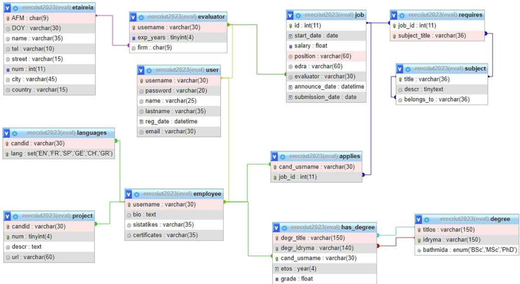
Εικόνα 1. Σχισιακό μοντέλο της βάσης δεδομένων
