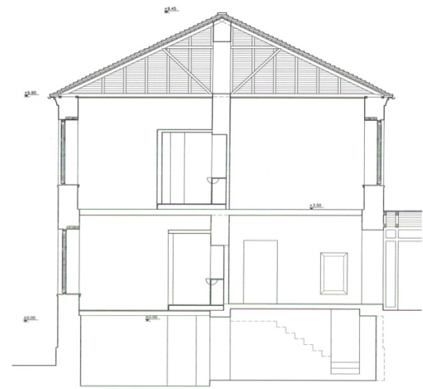
Κίτρο (Μίνα) Ζαχαρίου - Έντιν Παπαρρηγιού - ΠΡΟΤΑΣΗ Σχ.ΤΡ. ΟΙΚ.13 ΤΟΜΗ Θ κλ. 1:50
