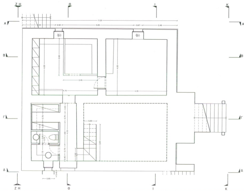
Κτίριο (Μπαγιά) Ζαχαριού - Έκτινών Πατισσαριού - ΠΡΩΤΑΞΗ Σχ.ΠΡ. ΟΙΚ.01 ΚΑΤΟΦΗ Α κλ. 1:50
