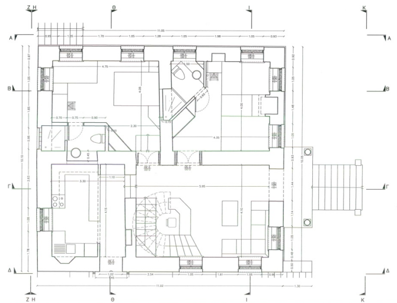
Κτίριο (Μπαγιά) Ζαχαριού - Έκτινών Πατισσαριού - ΠΡΩΤΑΞΗ Σχ.ΠΡ. ΟΙΚ.02 ΚΑΤΟΦΗ Β κλ. 1:50
