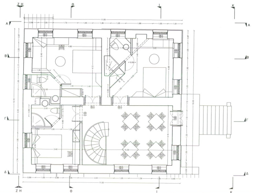
Κτίριο (Μπαγιά) Ζαχαριού - Έκτινών Πατισσαριού - ΠΡΩΤΑΞΗ Σχ.ΠΡ. ΟΙΚ.03 ΚΑΤΟΦΗ Γ κλ. 1:50
