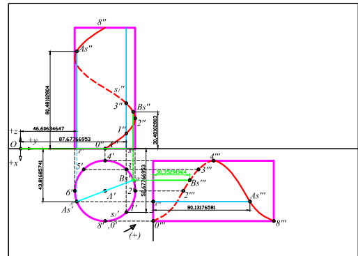
ΜΑΘΗΜΑ 4_ΑΣΚΗΣΗ 1_ΛΥΣΗ ΒΗΜΑ 3 ΒΟΗΘΗΤΙΚΟ ΣΧΗΜΑ ΑΠΟ ΜΟΝΓΕ ΓΙΑ ΤΟΝ ΠΡΟΣΔΙΟΡΙΣΜΟ ΤΩΝ ΣΗΜΕΙΩΝ ΕΠΑΦΗΣ ΕΛΙΚΑΣ ΜΕ ΟΡΙΚΕΣ ΓΕΝΕΤΕΙΡΕΣ ΚΥΛΙΝΔΡΟΥ ΣΤΗΝ ΑΞΟΝΟΜΕΤΡΙΑ
