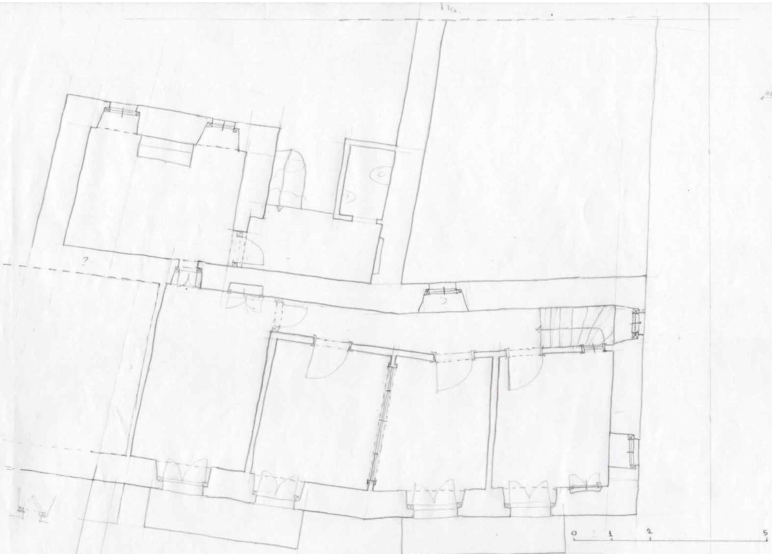
ΕΝΔΟΣ - ΠΕΝ - ΑΥ - ΧΑΛΑΝΔΡΙΤΣΑ - ΟΙΚΙΑ ΖΥΓΟΥΡΑΚΗ - ΚΑΤΟΨΗ Β - ΚΑΙΜΑΚΑ 1:50 - ΑΘΗΝΑΙΩΤΗΣ ΜΑΝΟΣ - 30.10.2020.
