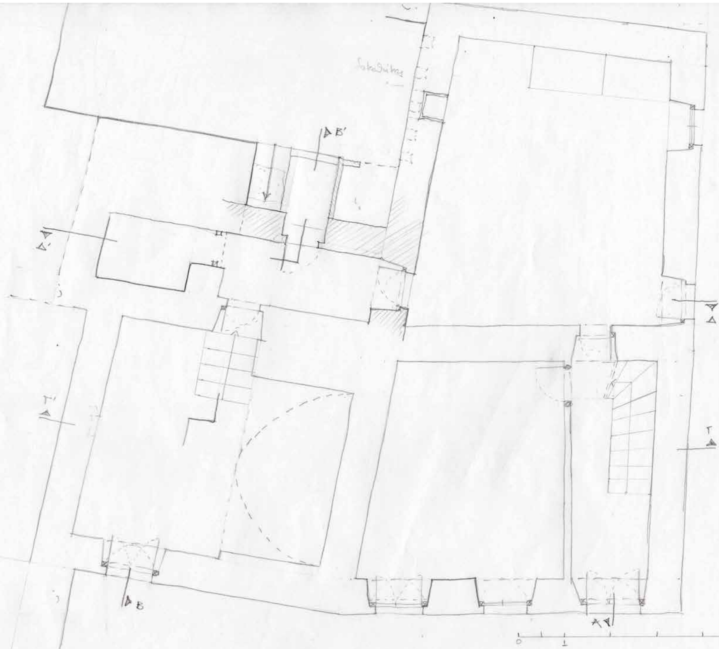
ΕΛΛΑΣ - ΠΕΛΛ - ΑΧ - ΧΑΛΑΝΔΡΙΤΣΑ - ΟΙΚΙΑ - ΖΥΓΟΥΡΑΚΗ ΚΑΤΟΨΗ Α ΚΛΙΜΑΚΑ 1:50 ΠΑΡΙΝΟΣ ΕΥΑΓΓΕΛΟΣ 30/10
