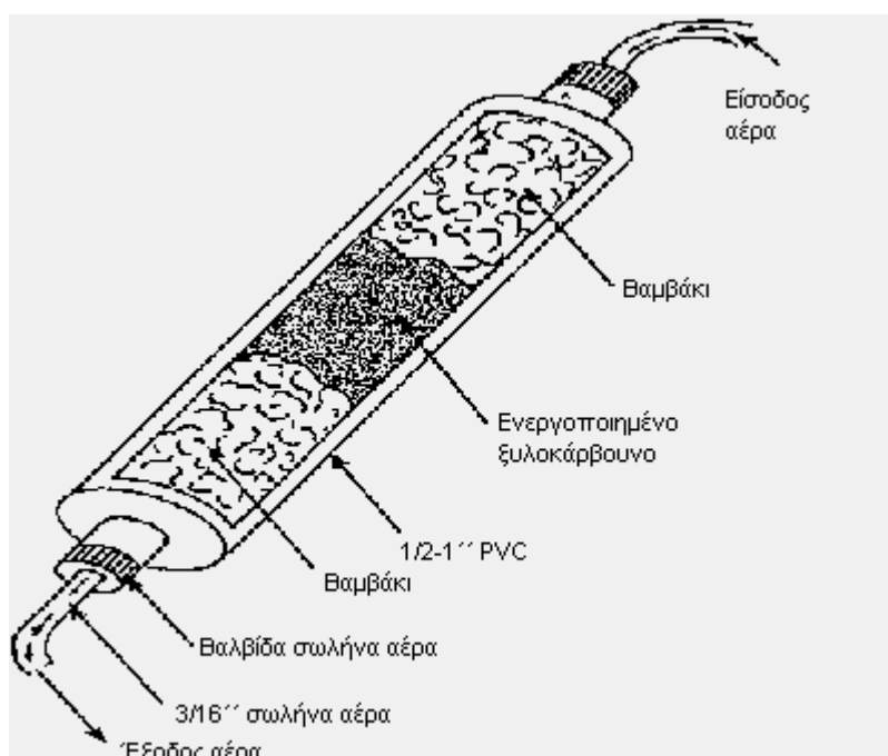
Σχήμα 31. Φίλτρο γραμμής παροχής αέρα.
