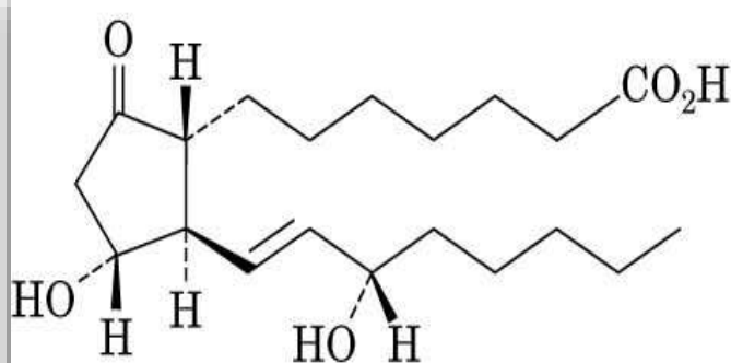
Prostaglandin E 1
