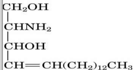
Sphingosine
