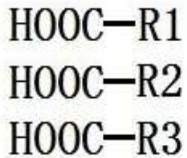
Λιπαρό οξύ
