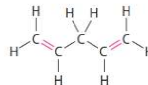
1,4-Πενταδιένιο (μη συζυγιακό)
