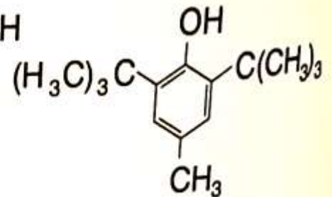
BHT
