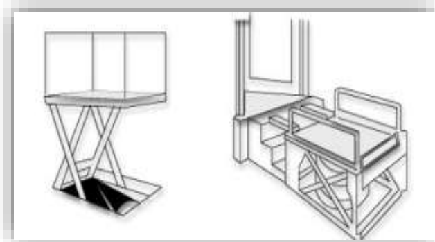
Εικόνα 94. Αναβατόρια κατακόρυφης κίνησης και κλίμακας (Ο.Σ.Κ., 2008)
