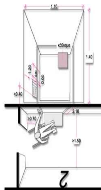
Εικόνα 81. Κάτοψη ανελκυστήρα (Ο.Σ.Κ., 2008)
