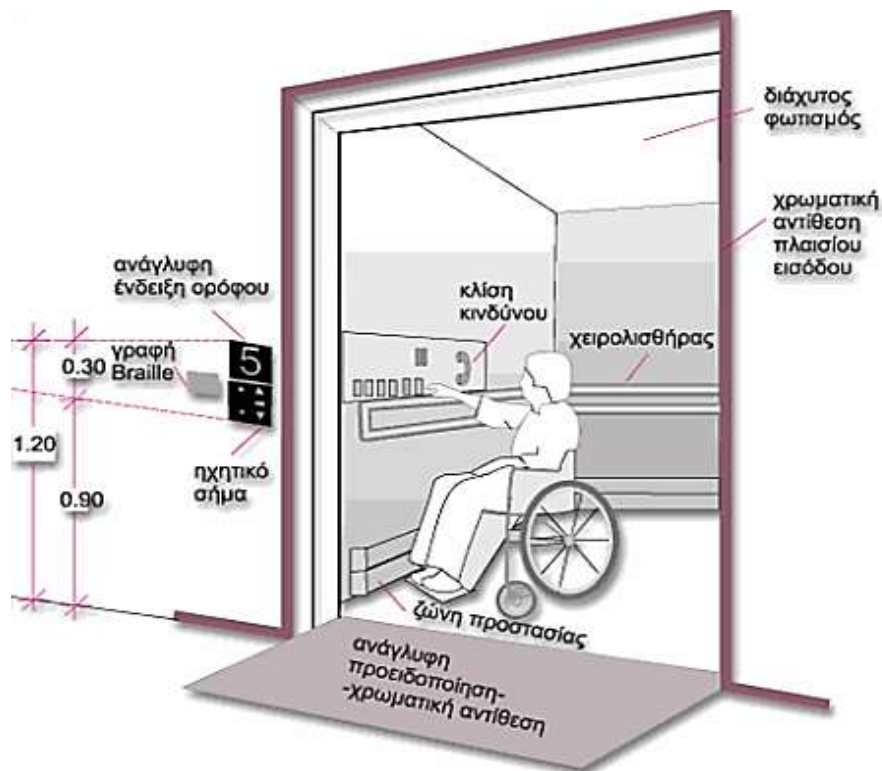
Εικόνα 77. Εξοπλισμός Θαλάμου (Ο.Σ.Κ., 2008)
