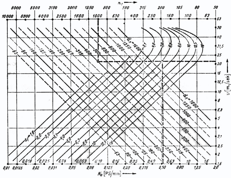
Σχήμα 14-11: Νομογράφημα ειδικής ισχύος N_0 για δερμάτινους μιάντες HG, s_f = s [1 - 10 / (d_1 / s)]
