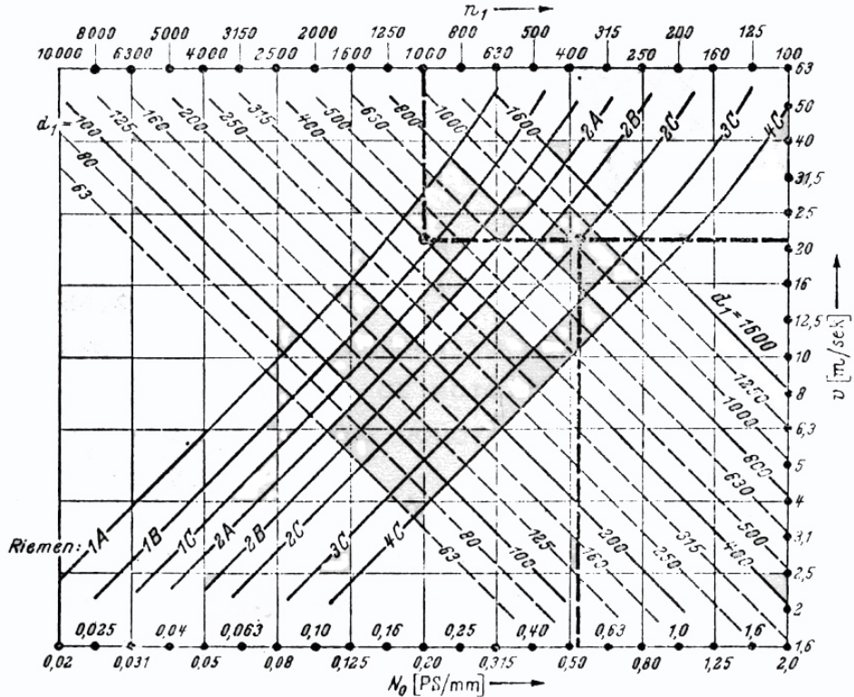
Σχήμα 14-12: Νομογράφημα ειδικής ισχύος N_0 για μιάντες Extremultus.
