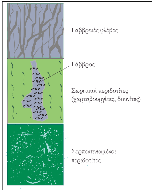
Εικ.3. Στρωματογραφική στήλη στην περιοχή του λατομικού χώρου ΤΕΡΝΑ Α.Ε.
