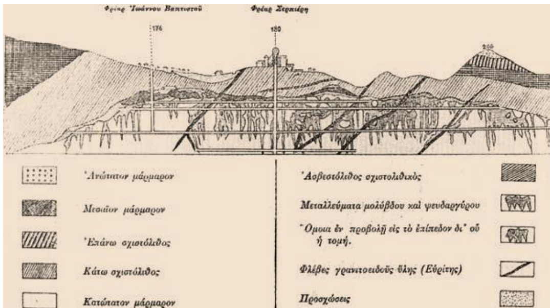
Εικ. 7. Τομή εδάφους σε ένα από τα κυριότερα φρεάτια μεταλλοφορίας της περιοχής Καμαρίζας.
