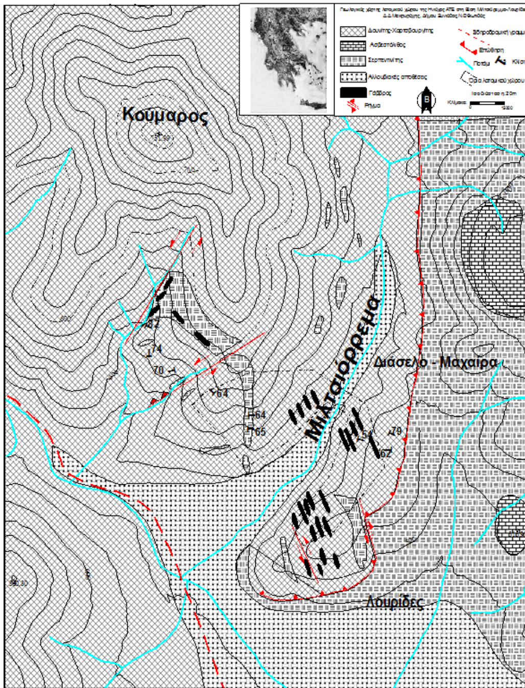
Εικ. 4. Γεωλογικός Χάρτης Περιοχής Μιλτσιόρρεμα-Λουρίδες (από Διπλ. Εργασία της Α. Αντωνέλου).
