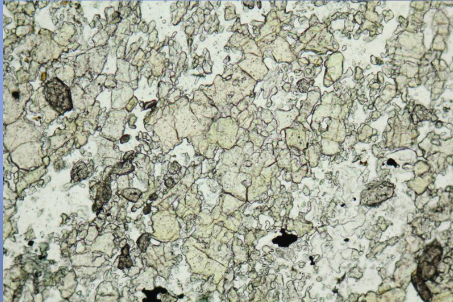
// Nicols , www.alexstrekeisen.it/immagini/meta/epidotii(7).jpg
