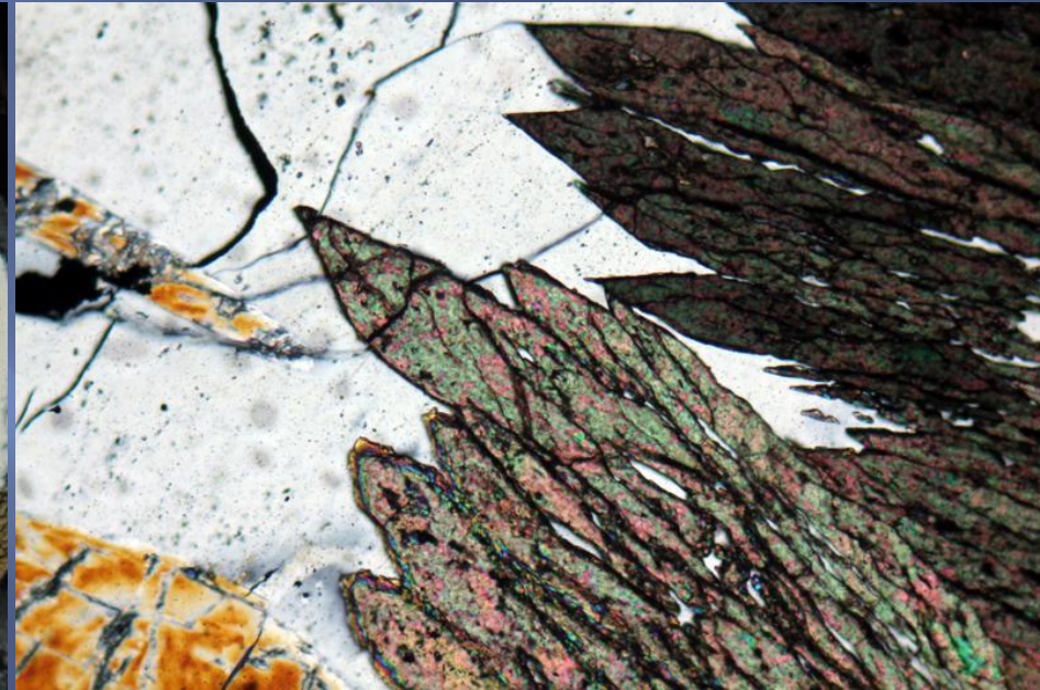
⊥ Nicols , http://www.alexstrekeisen.it/immagini/pluto/titaniteeee(3).jpg
