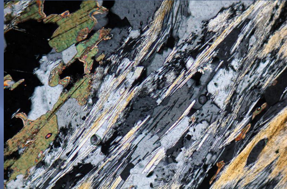
⊥ Nicols , http://www.alexstrekeisen.it/immagini/meta/fibrolite1682(17).jpg
