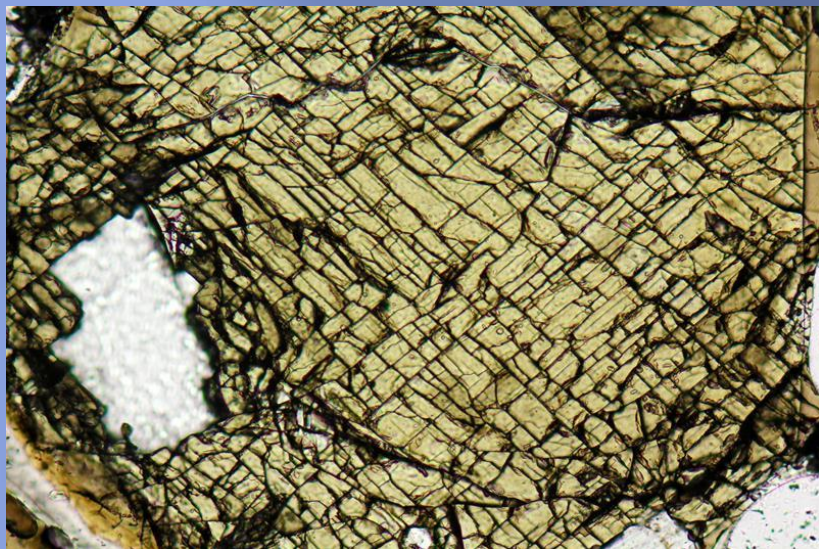
//Nicols , www.alexstrekeisen.it/immagini/vulc/pyroxene2020(17).jpg
