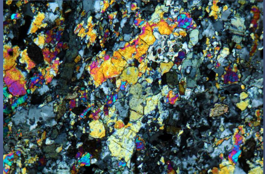
⊥ Nicols , www.alexstrekeisen.it/immagini/meta/epidotii(8).jpg
