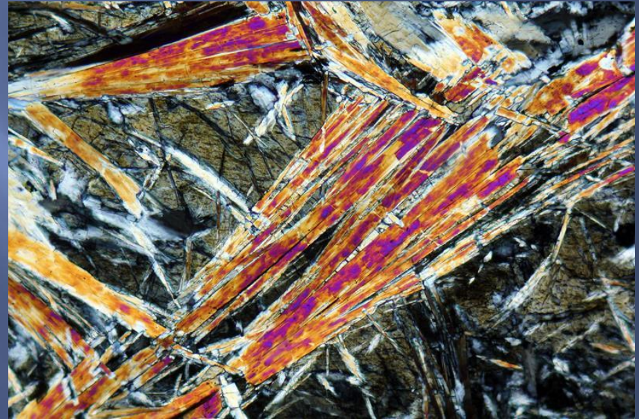
⊥ Nicols , www.alexstrekeisen.it/immagini/meta/actinolite(20).jpg
