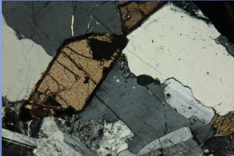
⊥ Nicols , http://www.alexstrekeisen.it/immagini/pluto/titaanite(4).jpg
