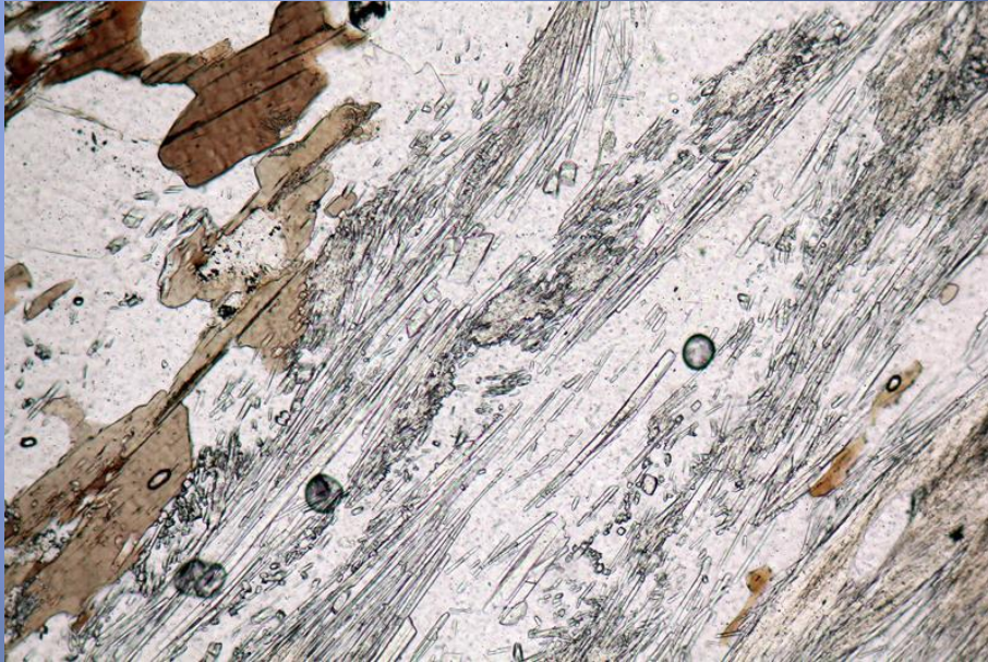
// Nicols , trekeisen.it/immagini/meta/fibrolite1682(16).jpg
