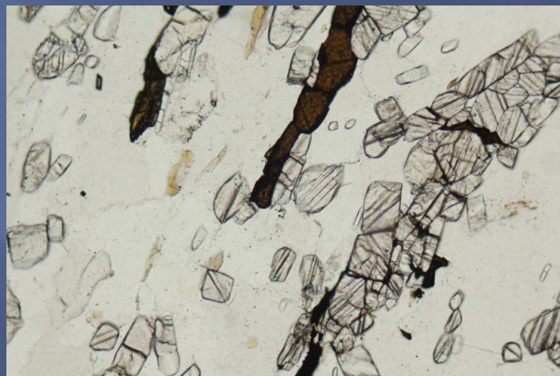
⊥ Nicols , http://www.alexstrekeisen.it/immagini/meta/fibrolite1682(17).jpg
