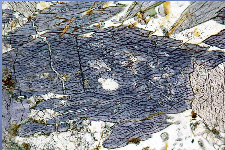
// Nicols , www.alexstrekeisen.it/immagini/meta/glaucofanemilos(25).jpg
