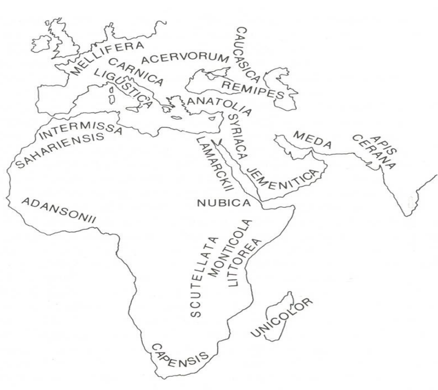
Φωτ.6. Περιοχές εξάπλωσης φυλών (ράτσες) της Apis mellifera .
