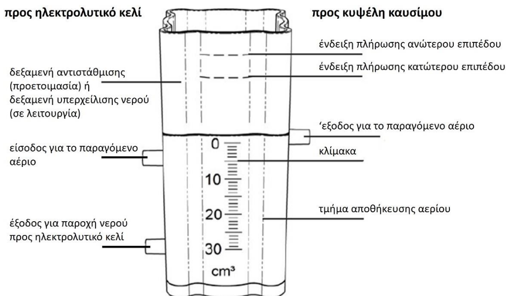
Σχήμα 5: Δεξαμενή για την αποθήκευση αερίου, h-tec [ ]
