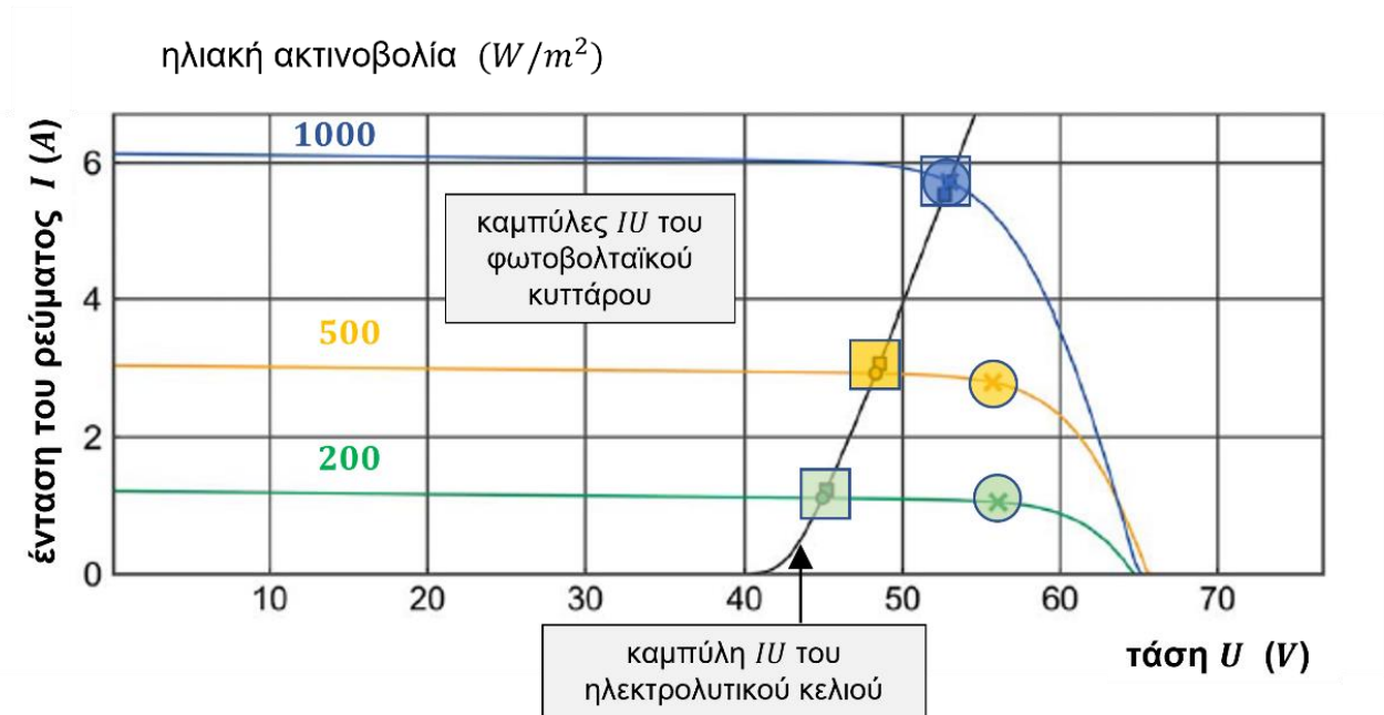
Σχήμα 3: Καμπύλες IU ενός φωτοβολταϊκού κυττάρου σε διαφορετικές συνθήκες φωτισμού επικαλυμμένες με την καμπύλη IU του ηλεκτρολυτικού κελιού [ ].
