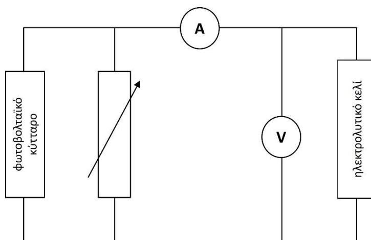
Σχήμα 7: Ηλεκτρικό κύκλωμα για την μελέτη της χαρακτηριστικής ( IU ) του ηλεκτρολυτικού κελιού με μη ελεγχόμενη πηγή τάσης
