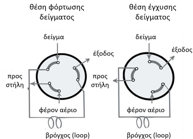
Σχήμα 5: Διάγραμμα ροής - Γενική λειτουργία της βαλβίδας έξι θυρών (youtube video Principle of a six port sampling valve )
