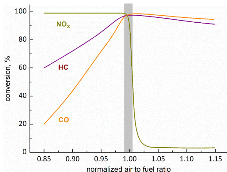
Σχήμα 2. Τυπικό διάγραμμα απόδοσης ενός Τριοδικού Καταλυτικού Μετατροπέα (TWC) για την μετατροπή των τριών κυριότερων ρύπων (HC, CO, \text{NO}_x ) ως συνάρτηση του λόγου αέρα/καύσιμο
