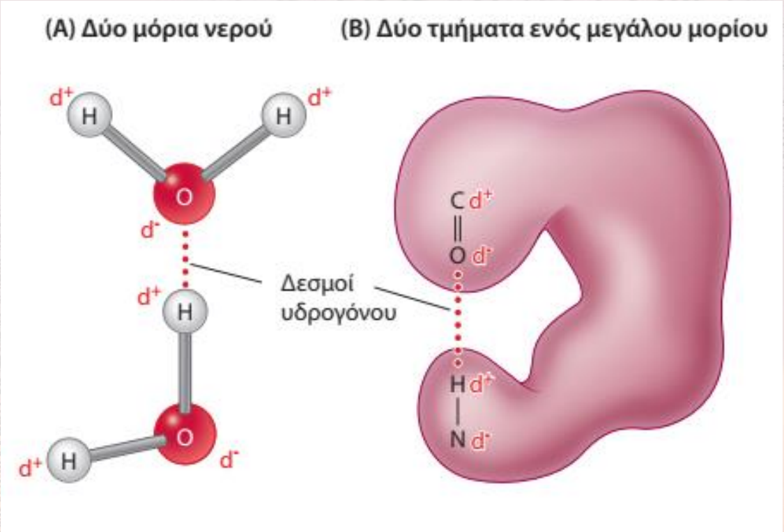
Εικόνα 2.10 Δεσμοί Υδρογόνου Μπορούν να Σχηματιστούν Μεταξύ ή Εντός των Μορίων (Α) Ένας δεσμός υδρογόνου μεταξύ δύο μορίων είναι μία έλξη μεταξύ ενός αρνητικού φορτίου σε ένα μόριο και του θετικού φορτίου σε ένα άτομο υδρογόνου του δεύτερου μορίου. (Β) Οι δεσμοί υδρογόνου μπορούν να σχηματιστούν μεταξύ διαφορετικών τμημάτων του ίδιου μεγάλου μορίου.
