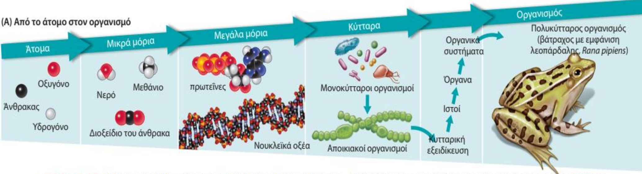
Εικόνα 1.10 Η Βιολογία Μελετάται σε Πολλά Επίπεδα Οργάνωσης (Α) Οι ιδιότητες της ζωής εμφανίζονται όταν το DNA και άλλα μόρια οργανώνονται στα κύτταρα, τα οποία αποτελούν δομικά στοιχεία των οργανισμών. (Β) Οι οργανισμοί υπάρχουν σε πληθυσμούς και αλληλεπιδρούν με άλλους πληθυσμούς για να σχηματίσουν κοινότητες οι οποίες αλληλεπιδρούν με το φυσικό περιβάλλον για να συνθέσουν τα πολλά οικοσυστήματα της βιόσφαιρας.
