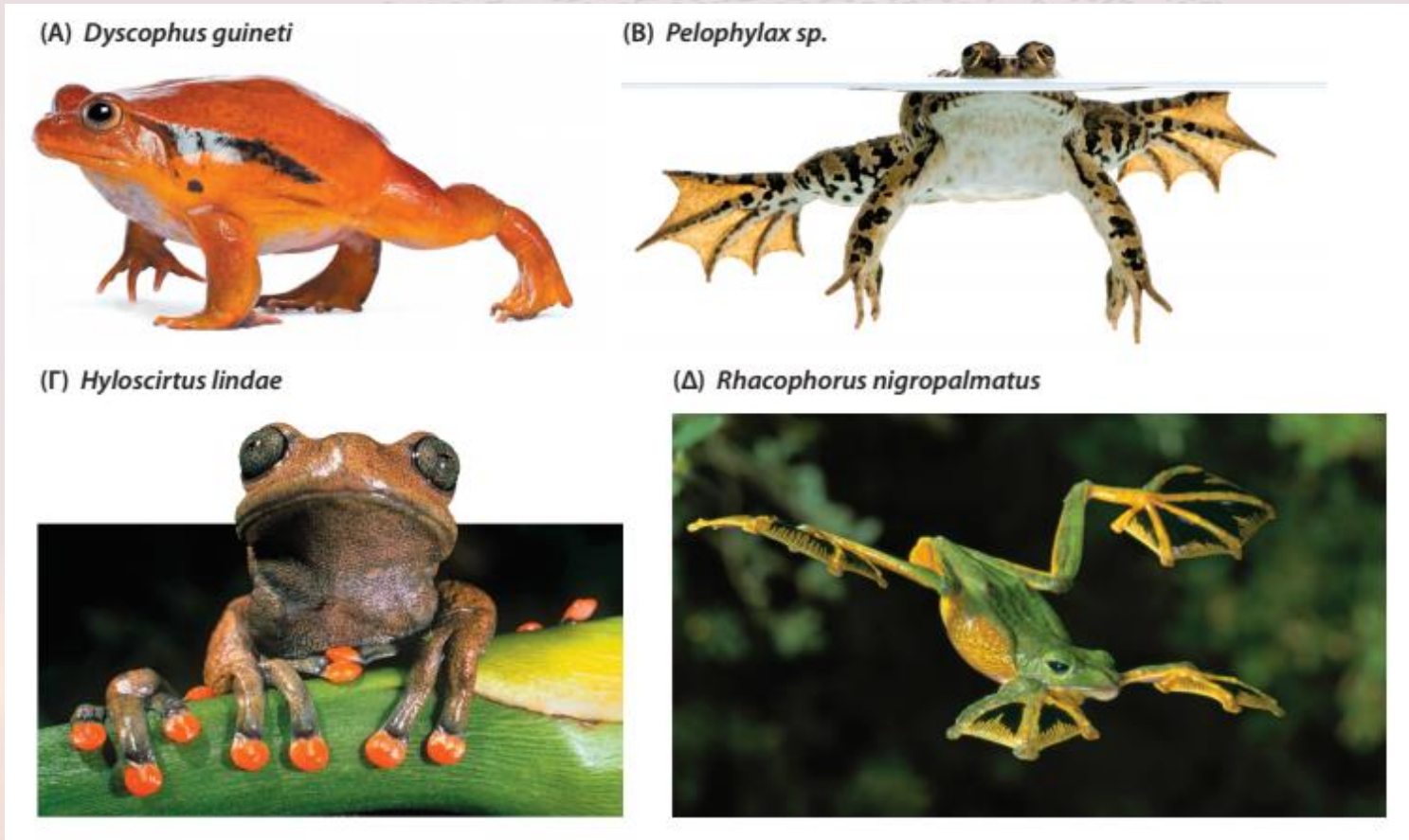
Εικόνα 1.7 Προσαρμογές στο Περιβάλλον Τα άκρα των βατράχων δείχνουν προσαρμογές στα διαφορετικά περιβάλλοντα κάθε είδους. (Α) Αυτός ο χερσαίος βάτραχος περπατάει στο έδαφος χρησιμοποιώντας τα κοντά του πόδια και τα δάκτυλα που μοιάζουν με μανταλάκια. (Β) Τα ενωμένα με μεμβράνη πίσω πόδια είναι εμφανή σε αυτό το άκρως υδρόβιο είδος βατράχου. (Γ) Αυτό το δενδρόβιο είδος έχει στα πόδια μαξιλαράκια, που αποτελούν προσαρμογές για αναρρίχηση. (Δ) Ένα διαφορετικό δενδρόβιο είδος έχει επεκτείνει το πλέγμα μεταξύ των δακτύλων, αυξάνοντας το εμβαδόν επιφανείας και επιτρέποντας στον βάτραχο να ολισθαίνει από δέντρο σε δέντρο.
