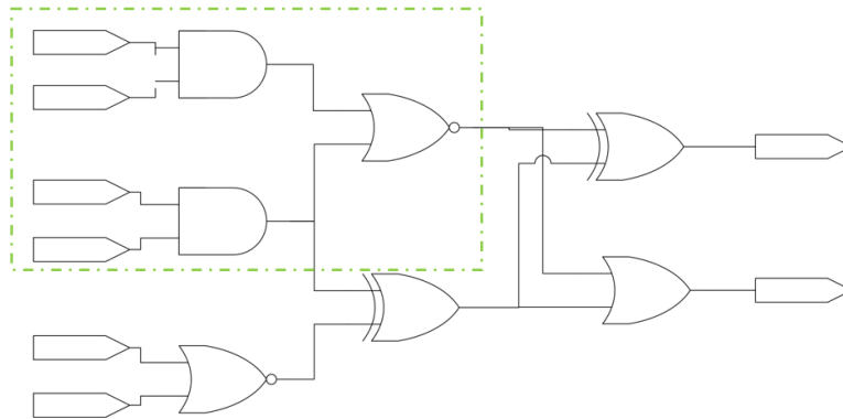
Σχήμα 1 Απλό κύκλωμα λογικών πυλών.
