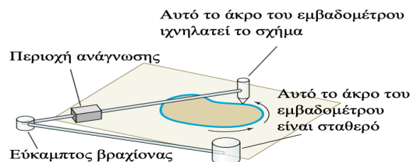
Σχήμα 3.82 Το εμβαδόμετρο είναι μια μηχανική συσκευή η οποία χρησιμοποιείται για τη μέτρηση των εμβαδών ακανόνιστων σχημάτων
