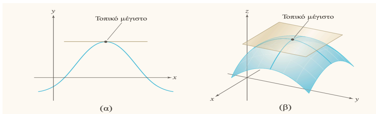
Σχήμα 2.29 Το γράφημα της συνάρτησης μοιάζει ολοένα και περισσότερο με το εφαπτόμενο επίπεδο στο σημείο P καθώς προχωράμε στην ολοένα και μεγαλύτερη μεγέθυνσή του.
