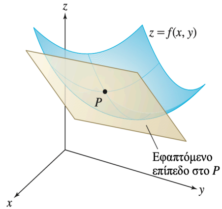
Σχήμα 2.22 Το εφαπτόμενο επίπεδο
