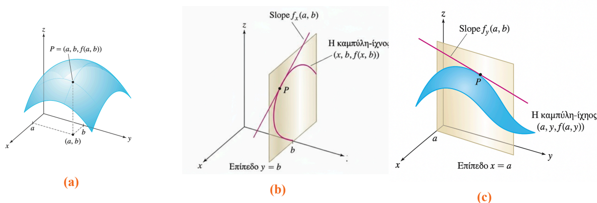
Σχήμα 2.19 Οι μερικές παράγωγοι και οι κλίσεις των καμπυλών-ίχνων
