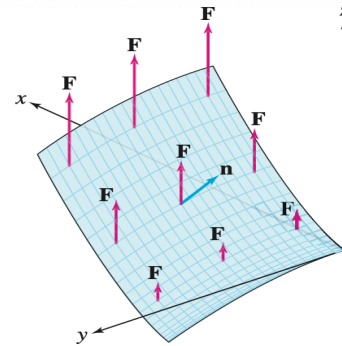
Σχήμα 3.69 Η επιφάνεια, με παραμέτρηση G(u, v) = (u^2, v, u^3 - v^2) , με κάθετα διανύσματα κατευθυνόμενα προς τα επάνω. Το διανυσματικό πεδίο F = \langle 0, 0, x \rangle έχει κατακόρυφη διεύθυνση.
