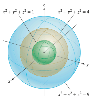
Σχήμα 2.11 Οι ισοσταθμικές επιφάνειες της συνάρτησης f(x, y, z) = x^2 + y^2 + z^2 είναι σφαίρες.
