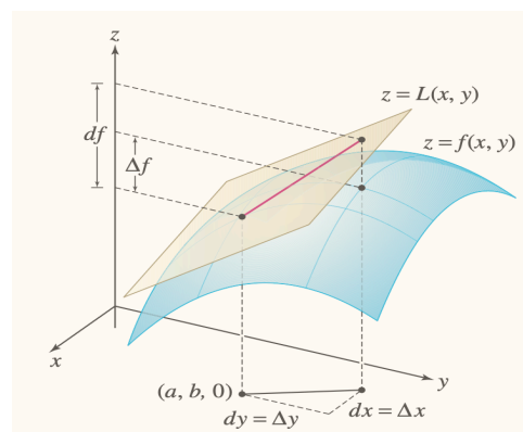
Σχήμα 2.26 Η γραφική παράσταση της συνάρτησης
