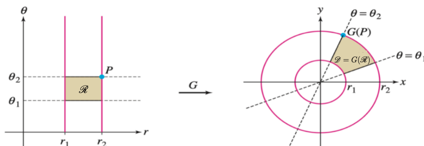
Σχήμα 2.75 Η απεικόνιση πολικών συντεταγμένων G(r, \theta) = (r \cos \theta, r \sin \theta) .
