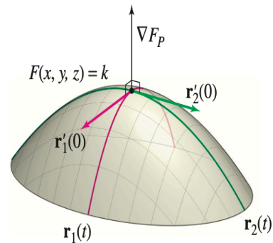
Σχήμα 3.18 Το διάνυσμα \nabla F_P είναι κάθετο στην επιφάνεια F(x, y, z) = k στο σημείο P .
