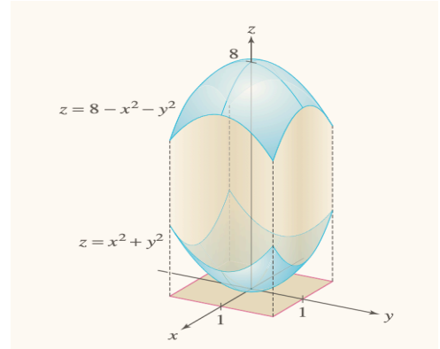
Σχήμα 2.49 Προσδιορισμός του όγκου ενός στερεού που βρίσκεται μεταξύ δύο παραβολοειδών πάνω από ένα τετράγωνο χωρίο
