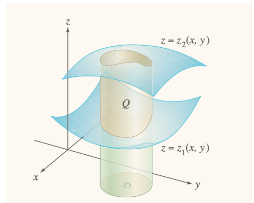
Σχήμα 2.50 Προσδιορισμός του όγκου ενός στερεού το οποίο περικλείεται μεταξύ δύο επιφανειών πάνω από ένα χωρίο D
