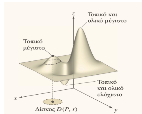
Σχήμα 2.28 Η συνάρτηση f(x,y) έχει ένα τοπικό μέγιστο στο P .
