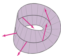
Η λωρίδα Möbius
