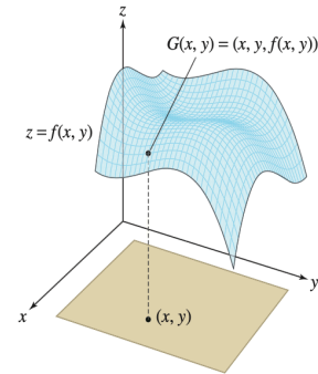
Σχήμα 3.60 Ο τρόπος παραμέτρησης του γραφήματος μιας συνάρτησης.
