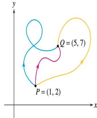
Σχήμα 3.48 Διαφορετικές διαδρομές από το (1, 2) στο (5, 7)
