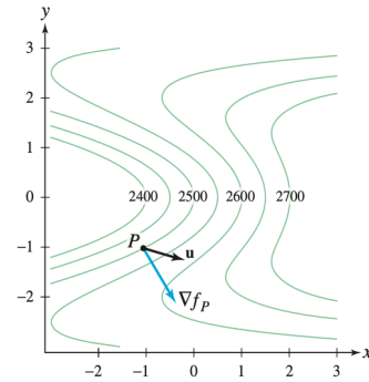
Σχήμα 3.17 Ισοσταθμικός χάρτης της συνάρτησης f(x, y) του Παραδείγματος 3.5.3.
