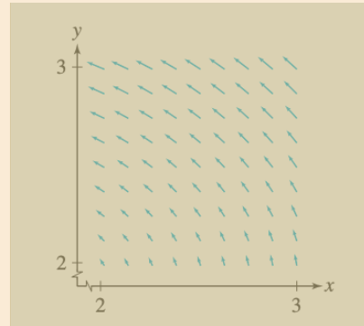
Σχήμα 3.85 Το διανυσματικό πεδίο \mathbf{F} = \langle xy - y^3, x^2 + y \rangle
