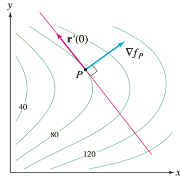
Σχήμα 3.16 Ισοσταθμικός χάρτης μιας συνάρτησης f(x, y) . Η κλίση της συνάρτησης στο σημείο P είναι ορθογώνια στην ισοσταθμική καμπύλη που διέρχεται από το P και «δείχνει» προς την κατεύθυνση της μέγιστης αύξησης της f(x, y) .
