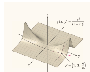
Σχήμα 2.17 Οι κλίσεις των εφαπτόμενων ευθειών στις καμπύλες-ίχνη στο σημείο P είναι οι g_x(1,3) και g_y(1,3)
