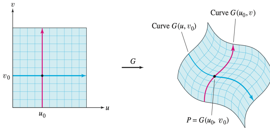
Σχήμα 3.61 Πλεγματικές καμπύλες.
