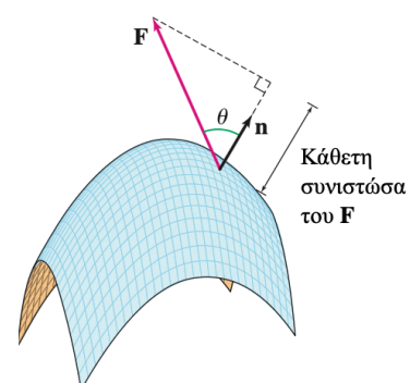
Σχήμα 3.68 Η κάθετη συνιστώσα ενός διανύσματος σε
