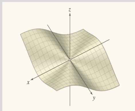
Σχήμα 2.15 Η γραφική παράσταση της συνάρτησης f(x,y) = \frac{xy^2}{x^2 + y^2} .
