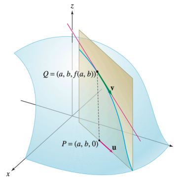
Σχήμα 3.14 Η παράγωγος κατά κατεύθυνση D_{\mathbf{u}}f(a, b) είναι η κλίση της εφαπτόμενης ευθείας στην καμπύλη-ίχνος στο σημείο Q στο κατακόρυφο επίπεδο που διέρχεται από το σημείο P στην κατεύθυνση του διανύσματος \mathbf{u} . Το διάνυσμα \mathbf{v} = \langle h, k, D_{\mathbf{u}}f(P) \rangle είναι παράλληλο σε αυτή την εφαπτόμενη ευθεία.
