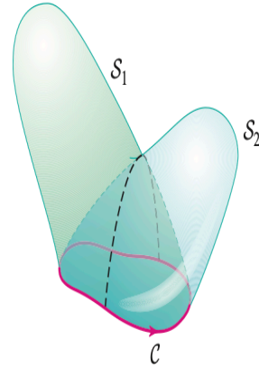
Σχήμα 3.91 Οι επιφάνειες S_1 και S_2 έχουν την ίδια καμπύλη ως προσανατολισμένο σύνορο
