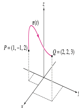
Σχήμα 3.47 Μια τυχαία διαδρομή από το σημείο (1, -1, 2) στο (2, 2, 3)
