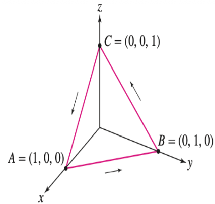
Σχήμα 3.37 Το τρίγωνο είναι κατά τμήματα λείο: Είναι η ένωση των τριών πλευρών του, κάθε μία από τις οποίες είναι λεία
