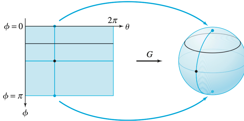
Σχήμα 3.59 Η παραμέτρηση με τη βοήθεια των σφαιρικών συντεταγμένων συνίσταται στο «τύλιγμα» του ορθογωνίου πάνω στη σφαίρα. Η πάνω και η κάτω πλευρά του ορθογωνίου «καταρρέουν» σε ένα σημείο καθώς αντιστοιχούνται στον βόρειο και νότιο πόλο της σφαίρας αντιστοίχως.
