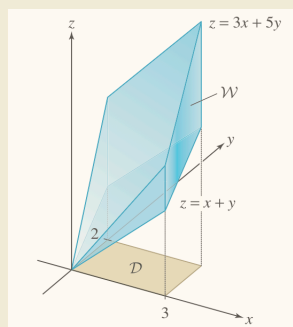
Σχήμα 2.58 Η περιοχή \mathcal{W} περικλείεται μεταξύ των επιπέδων z = x + y και z = 3x + 5y και εκτείνεται πάνω από το χωρίο \mathcal{D} = [0, 3] \times [0, 2]
