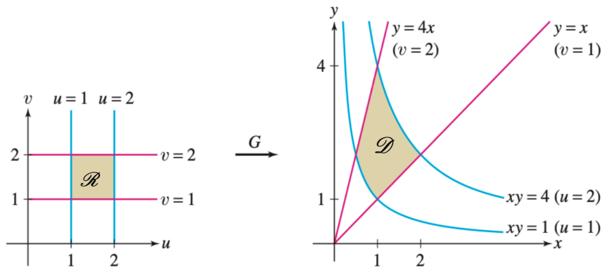
Σχήμα 2.78 Η απεικόνιση G(u, v) = (uv^{-1}, uv) .
