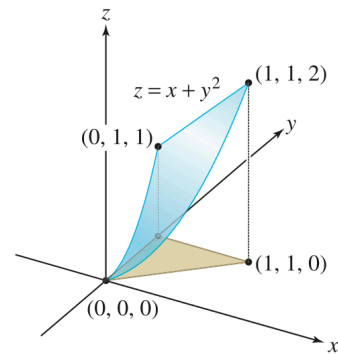
Σχήμα 3.66 Η επιφάνεια z = x + y^2 που βρίσκεται πάνω από το χωρίο που ορίζεται από τις ανισώσεις 0 \leq x \leq y και 0 \leq y \leq 1 .
