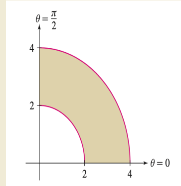
Σχήμα 2.67 Το ένα τέταρτο ενός δακτυλίου που ορίζεται από τις ανισώσεις 0 \leq \theta \leq \frac{\pi}{2} , 2 \leq r \leq 4 .
