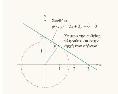
Σχήμα 2.35 Εύρεση του ελαχίστου της συνάρτησης f(x, y) = \sqrt{x^2 + y^2} πάνω στην ευθεία 2x + 3y = 6 .
