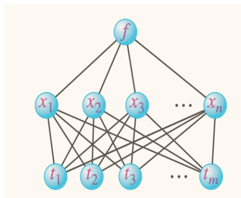
Σχήμα 2.20 Σκαρίφημα με το οποίο μπορούμε να παρατηρούμε τις εξαρτήσεις μεταξύ των μεταβλητών.
