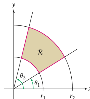
Σχήμα 2.66 Πολικές συντεταγμένες
