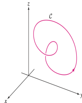
Σχήμα 3.49 Το επικαμπύλιο ολοκλήρωμα ενός συντηρητικού διανυσματικού πεδίου σε μια κλειστή διαδρομή είναι μηδέν
