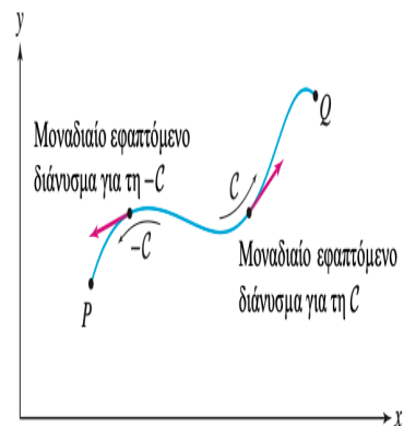
Σχήμα 3.36 Η καμπύλη μεταξύ των σημείων P και Q μπορεί να προσανατολιστεί με δύο διαφορετικούς τρόπους
