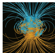
Σχήμα 2.65 Οι σφαιρικές συντεταγμένες χρησιμοποιούνται στη μελέτη μαθηματικών μοντέλων του γήινου μαγνητικού πεδίου. Στην εικόνα, που έχει δημιουργηθεί με τη βοήθεια προσομοίωσης σε ηλεκτρονικό υπολογιστή με βάση το μοντέλο Glatzmaier-Roberts, απεικονίζονται οι μαγνητικές δυναμικές γραμμές που εισέρχονται (με μπλε χρώμα) και εξέρχονται (με κίτρινο χρώμα) από τη Γη.
