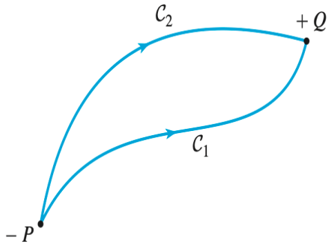
Σχήμα 3.90 Δύο διαδρομές με το ίδιο σύνολο Q - P
