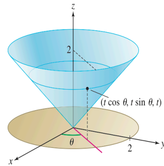
Σχήμα 3.65 Το τμήμα S του κώνου x^2 + y^2 = z^2 που βρίσκεται πάνω από τον δίσκο x^2 + y^2 \leq 4 .
