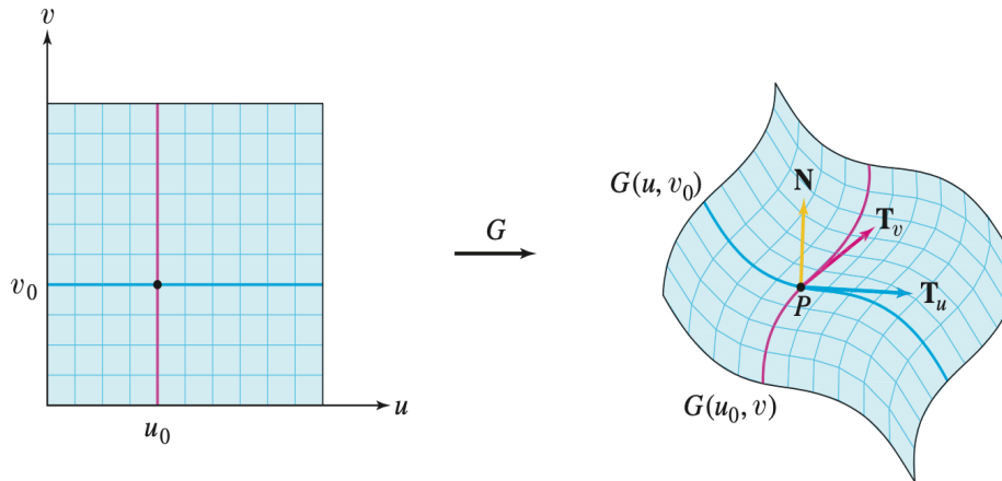
Σχήμα 3.62 Τα διανύσματα T_u και T_v είναι εφαπτόμενα στις πλεγματικές καμπύλες που διέρχονται από το P = G(u_0, v_0) .
