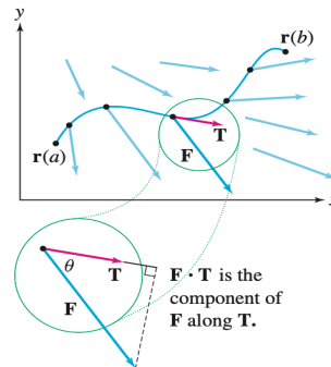
Σχήμα 3.34 Το επικαμπύλιο ολοκλήρωμα του πεδίου \mathbf{F} κατά μήκος της καμπύλης C είναι ίσο με το επικαμπύλιο ολοκλήρωμα της εφαπτομενικής συνιστώσας του πεδίου \mathbf{F} πάνω στην καμπύλη.
