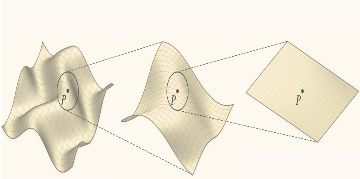
Σχήμα 2.25 Το γράφημα της συνάρτησης μοιάζει ολοένα και περισσότερο με το εφαπτόμενο επίπεδο στο σημείο P καθώς προχωράμε στην ολοένα και μεγαλύτερη μεγέθυνσή του.
