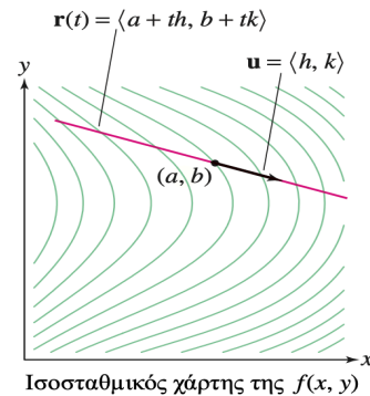
Σχήμα 3.13 Η παράγωγος κατά κατεύθυνση D_{\mathbf{u}}f(a, b) δείχνει τον ρυθμό μεταβολής της συνάρτησης f κατά μήκος της ευθείας που διέρχεται από το σημείο P έχοντας διάνυσμα κατεύθυνσης \mathbf{u} .
