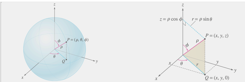
Σχήμα 3.57 Οι σφαιρικές συντεταγμένες (\rho, \theta, \phi)
