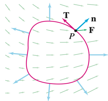
Σχήμα 3.83 Η ροή του πεδίου \mathbf{F} είναι ίση με το ολοκλήρωμα της κάθετης συνιστώσας \mathbf{F} \cdot \mathbf{n} κατά μήκος της καμπύλης.
