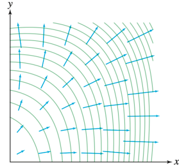
Σχήμα 3.21 Ένα συντηρητικό διανυσματικό πεδίο προκύπτει από την κλίση μιας βαθμωτής συνάρτησης δυναμικού και επομένως θα είναι ορθογώνιο προς τις ισοσταθμικές καμπύλες αυτής της συνάρτησης.
