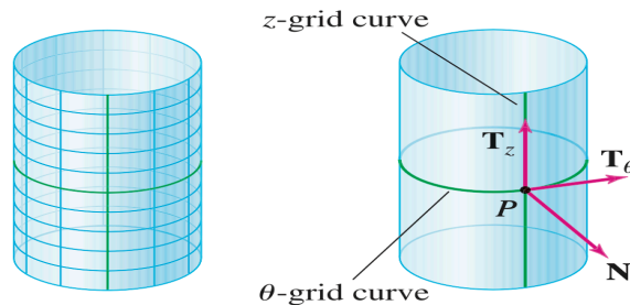
Σχήμα 3.63 Πλεγματικές καμπύλες του κυλίνδρου.
