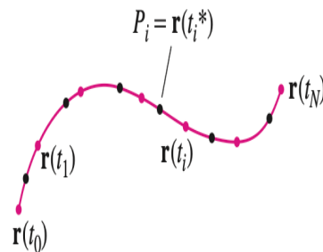
Σχήμα 3.29 Διαμέριση της παραμετρικής καμπύλης \mathbf{r}(t) .
