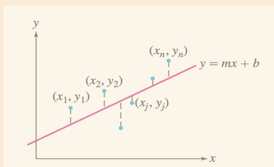
Σχήμα 2.34 Η βέλτιστη ευθεία ελαχίστων τετραγώνων ελαχιστοποιεί το άθροισμα των τετραγώνων των κατακόρυφων αποστάσεων μεταξύ των δεδομένων σημείων και της ευθείας.
