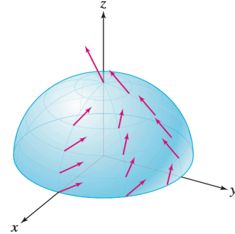
Σχήμα 3.70 Το διανυσματικό πεδίο \mathbf{F} = \langle z, x, 1 \rangle .
