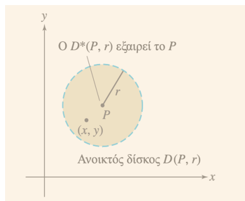
Σχήμα 2.12 Ο ανοικτός δίσκος D(P, r) αποτελείται από το σύνολο των σημείων (x, y) που βρίσκονται σε απόσταση μικρότερη του r από το σημείο P . Σε αυτόν δεν συμπεριλαμβάνεται ο συνοριακός κύκλος..
