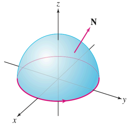
Σχήμα 3.88 Το άνω ημισφαίριο με προσανατολισμένη συνοριακή καμπύλη
