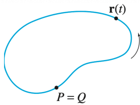
(a) Η κυκλοφορία κατά μήκος μιας κλειστής διαδρομής
