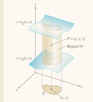
Σχήμα 2.57 Το σημείο P = (x, y, z) ανήκει στη z -απλή περιοχή \mathcal{W} αν (x, y) \in \mathcal{D} και z_1(x, y) \leq z \leq z_2(x, y)
