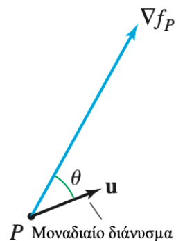
Σχήμα 3.15 D_{\mathbf{u}}f(P) = \|\nabla f_P\| \cos \theta
