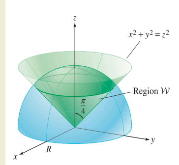
Σχήμα 2.72 Το χωνάκι ενός παγωτού ορίζεται από τις ανισώσεις 0 \leq \rho \leq R , 0 \leq \phi \leq \frac{\pi}{4}
