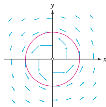
(b) Το πεδίο δίνης (ή πεδίο καταβόθρα)
