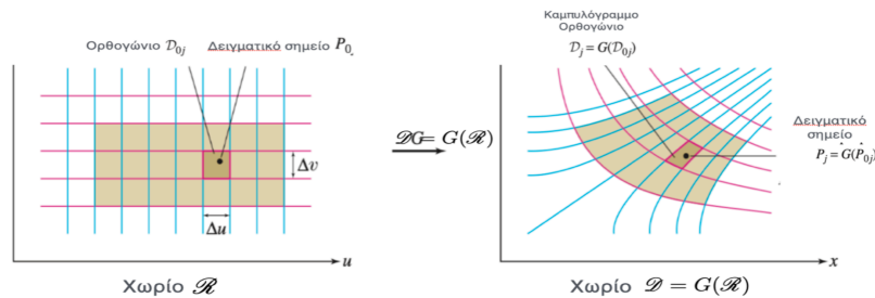
Σχήμα 2.74 Η G απεικονίζει ένα ορθογώνιο πλέγμα \mathcal{R} σε ένα καμπυλωμένο πλέγμα \mathcal{D} .
