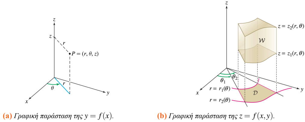
Σχήμα 2.69 Κυλινδρικές συντεταγμένες και περιγραφή χωρίου
