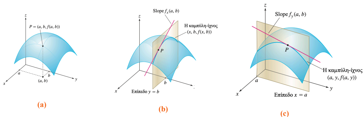
Σχήμα 2.18 Οι μερικές παράγωγοι και οι κλίσεις των καμπυλών-ίχνων
