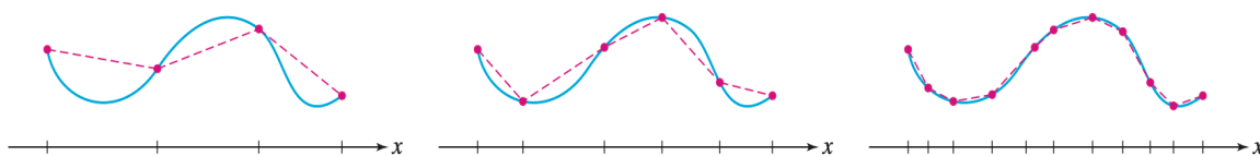
Σχήμα 3.26 Οι πολυγωνικές προσεγγίσεις βελτιώνονται καθώς μειώνεται η νόρμα της διαμέρισης.
