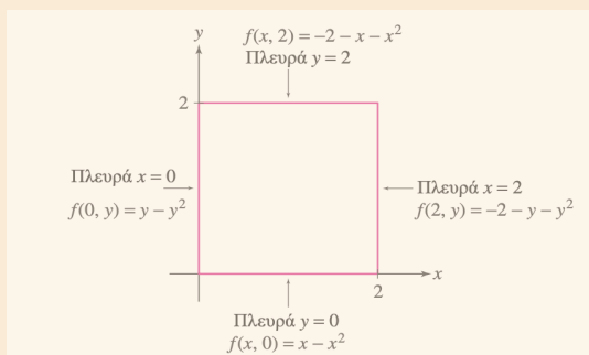
Σχήμα 2.33 Οι τύποι της συνάρτησης f(x,y) = x + y - x^2 - y^2 - xy στο σύνορο του τετραγώνου 0 \leq x \leq 2, 0 \leq y \leq 2
