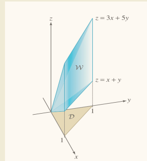
Σχήμα 2.59 Η περιοχή \mathcal{W} περικλείεται μεταξύ των επιπέδων z = x + y και z = 3x + 5y και εκτείνεται πάνω από το τριγωνικό χωρίο \mathcal{D} .
