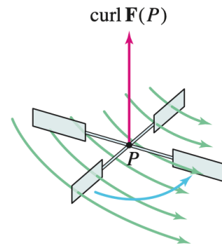
Σχήμα 3.20 Το διάνυσμα \operatorname{curl} \mathbf{F}(P) σχετίζεται με την περιστροφή ενός ρευστού.
