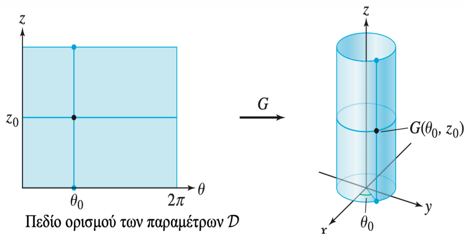
Σχήμα 3.56 Η παραμέτρηση ενός κυλίνδρου με τη βοήθεια των κυλινδρικών συντεταγμένων συνίσταται στο «τύλιγμα» ενός ορθογωνίου γύρω από έναν κύλινδρο.
