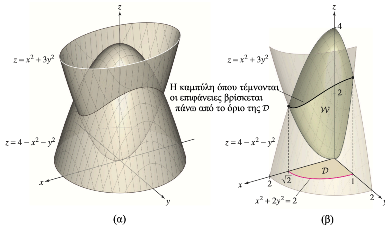
Σχήμα 2.60 Το στερεό που περιορίζεται μεταξύ των παραβολοειδών z = 4 - x^2 - y^2 και z = x^2 + 3y^2 φαίνεται στο (α). Η περιοχή στην οποία λαμβάνει χώρα η ολοκλήρωση φαίνεται στο (β).
