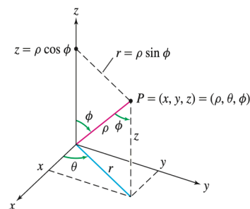
Σχήμα 2.71 Σφαιρικές συντεταγμένες
