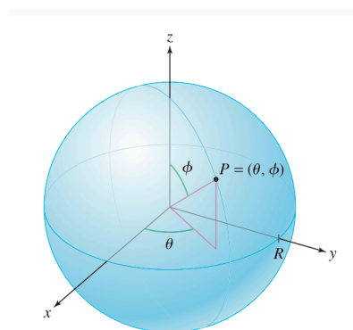
Σχήμα 3.58 Σφαιρικές συντεταγμένες για τα σημεία μιας σφαίρας ακτίνας R
