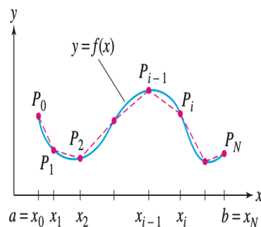
Σχήμα 3.25 Μια πολυγωνική προσέγγιση L της y = f(x) .
