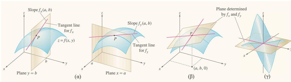
Σχήμα 2.23 Είναι το επίπεδο που προσδιορίζεται από τις f_x και f_y εφαπτόμενο στο γράφημα της συνάρτησης;
