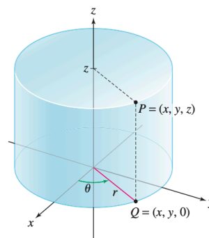
Σχήμα 3.55 Το σημείο P έχει κυλινδρικές συντεταγμένες (r, \theta, z)
