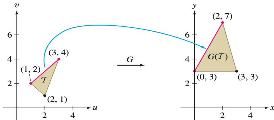
Σχήμα 2.77 Η απεικόνιση G(u, v) = (2u - v, u + v) .
