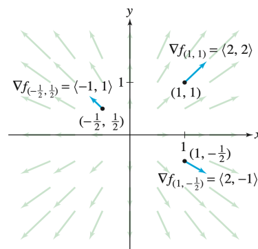
Σχήμα 3.10 Τα διανύσματα της κλίσης για τη συνάρτηση f(x, y) = x^2 + y^2 σε διάφορα σημεία (τα διανύσματα δεν είναι σχεδιασμένα έτσι ώστε να διατηρούν την κλίμακα).
