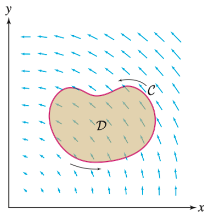
Σχήμα 3.81 Το επικαμπύλιο ολοκλήρωμα του διανυσματικού πεδίου \langle -y/2, x/2 \rangle πάνω στην καμπύλη C είναι ίσο με το εμβαδόν του χωρίου D το οποίο περικλείεται από την καμπύλη C .
