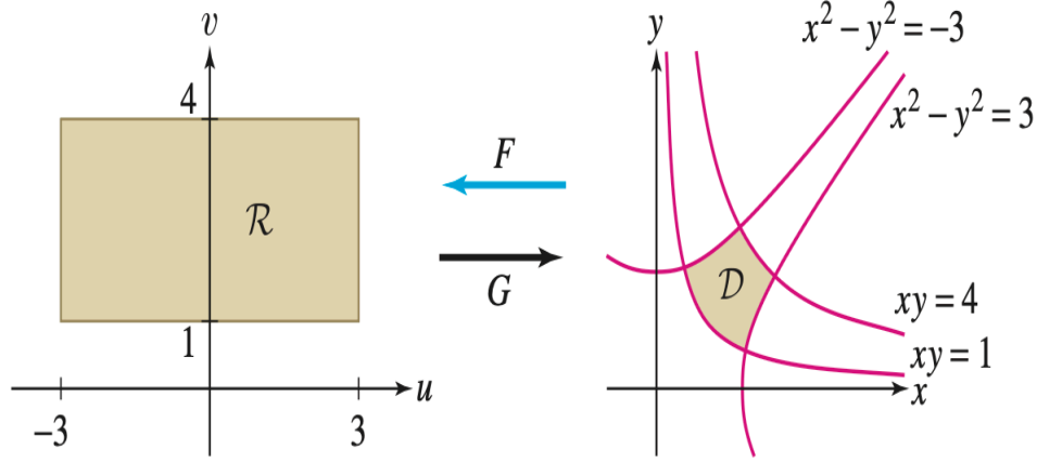
Σχήμα 2.79 Η απεικόνιση F έχει την αντίστροφη κατεύθυνση.
