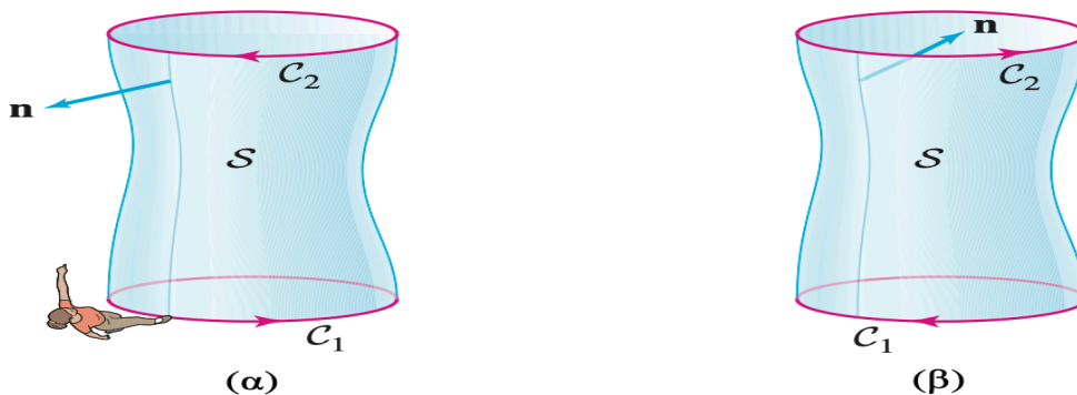
Σχήμα 3.87 Οι προσανατολισμοί της συνοριακής καμπύλης \partial S για καθέναν από τους δύο πιθανούς προσανατολισμούς της επιφάνειας S .
