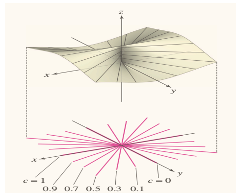
Σχήμα 2.14 Η γραφική παράσταση και ο ισοσταθμικός χάρτης της συνάρτησης f(x,y) = \frac{x^2}{x^2 + y^2} .
