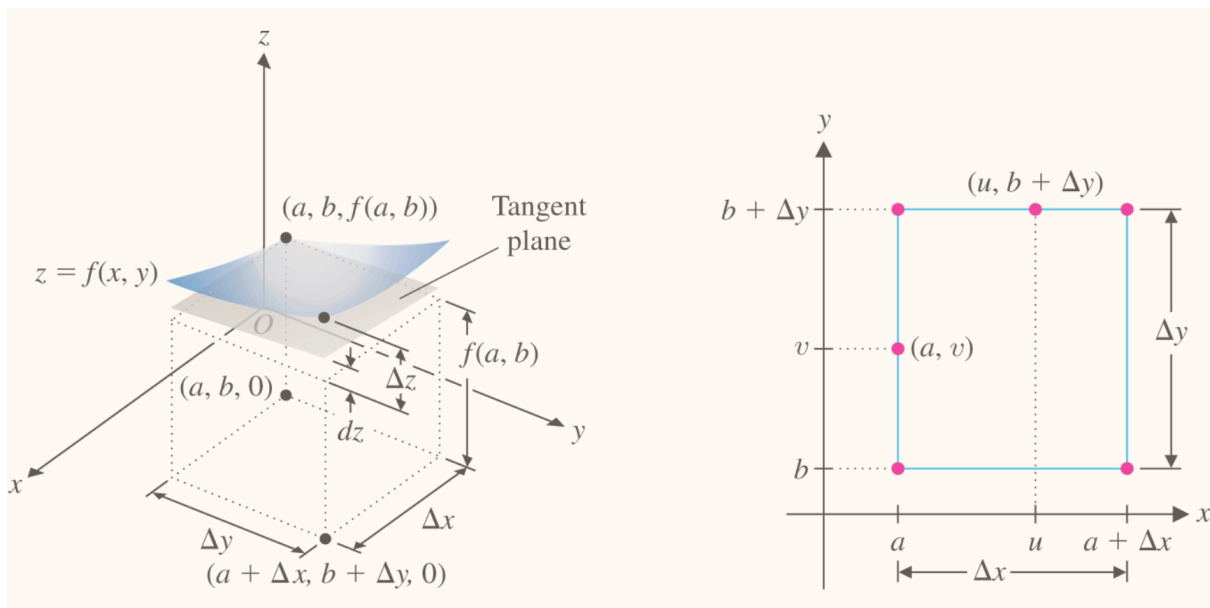
Σχήμα 2.24 Είναι το επίπεδο που προσδιορίζεται από τις f_x και f_y εφαπτόμενο στο γράφημα της συνάρτησης;
