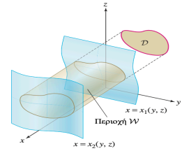
Σχήμα 2.61 Το χωρίο \mathcal{D} είναι η προβολή του στερεού \mathcal{W} πάνω στο επίπεδο yz .
