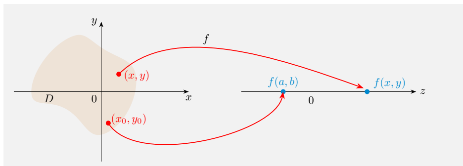
Σχήμα 2.1 Απεικόνιση του f : D \subseteq \mathbb{R}^2 \rightarrow \mathbb{R}
