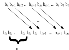
m θέσεων Αριθμητική Ολίσθηση Δεξιά
