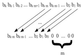
m θέσεων Λογική Ολίσθηση Αριστερά
