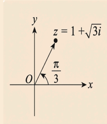
Σχήμα 4.13 Πολικές συντεταγμένες
