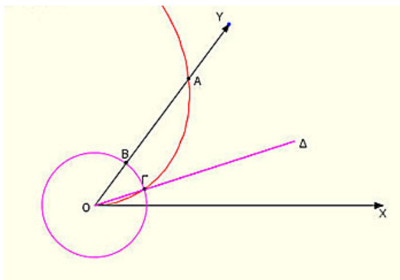
Σχήμα 1.3 Η τριχοτόμηση οξείας γωνίας του Αρχιμήδη.
