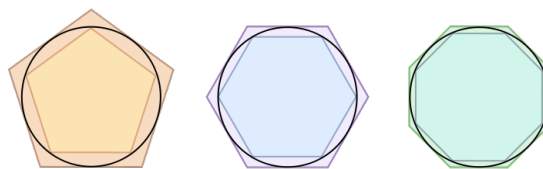
Σχήμα 1.4 Η προσέγγιση του Αρχιμήδη στον υπολογισμό του \pi .
