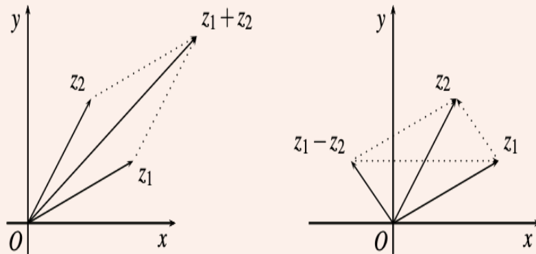
Σχήμα 4.11 Κανόνας του παραλληλογράμμου
