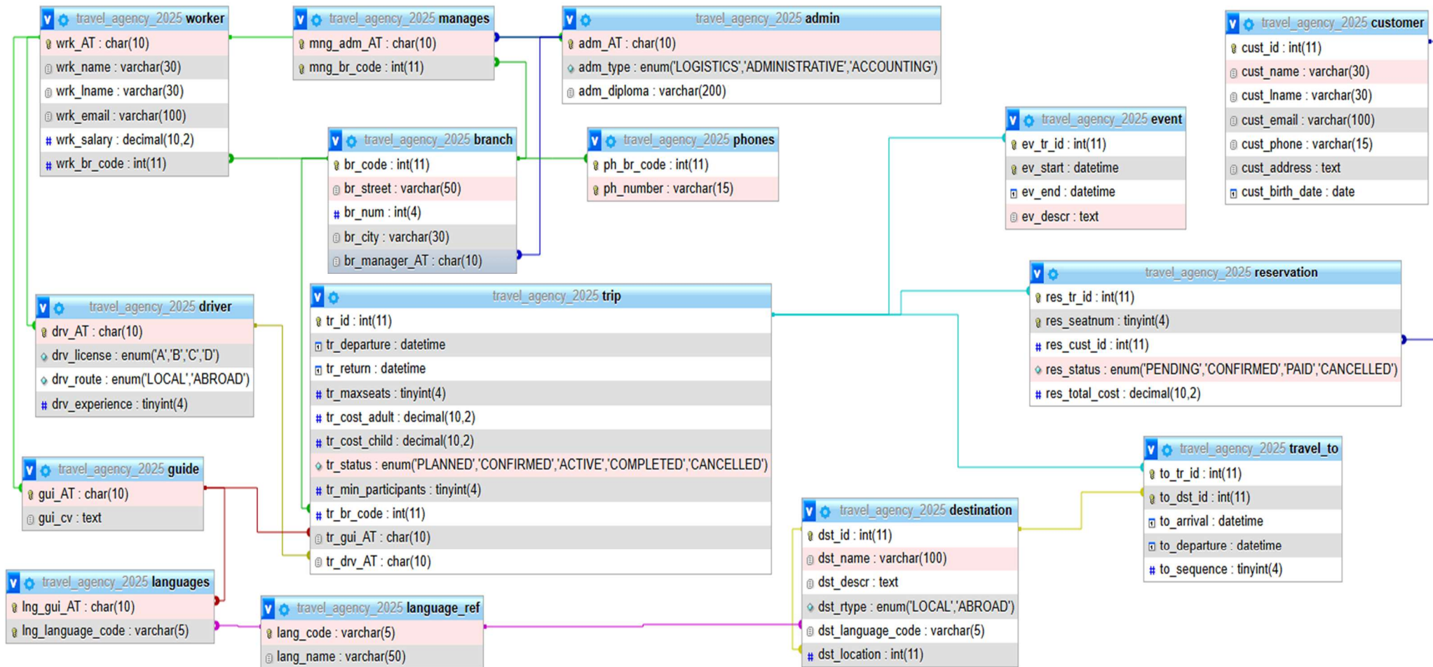
Εικόνα 1. Σχεσιακό μοντέλο της βάσης δεδομένων
