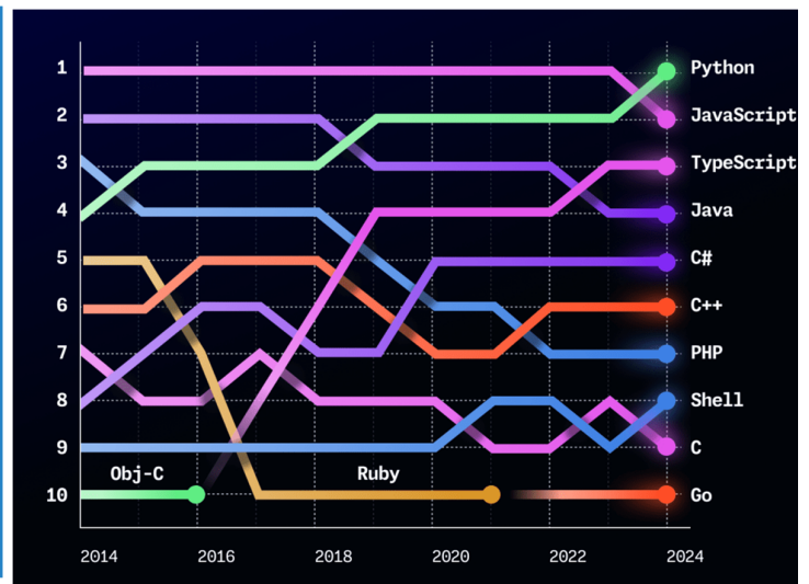
Github (2024)
