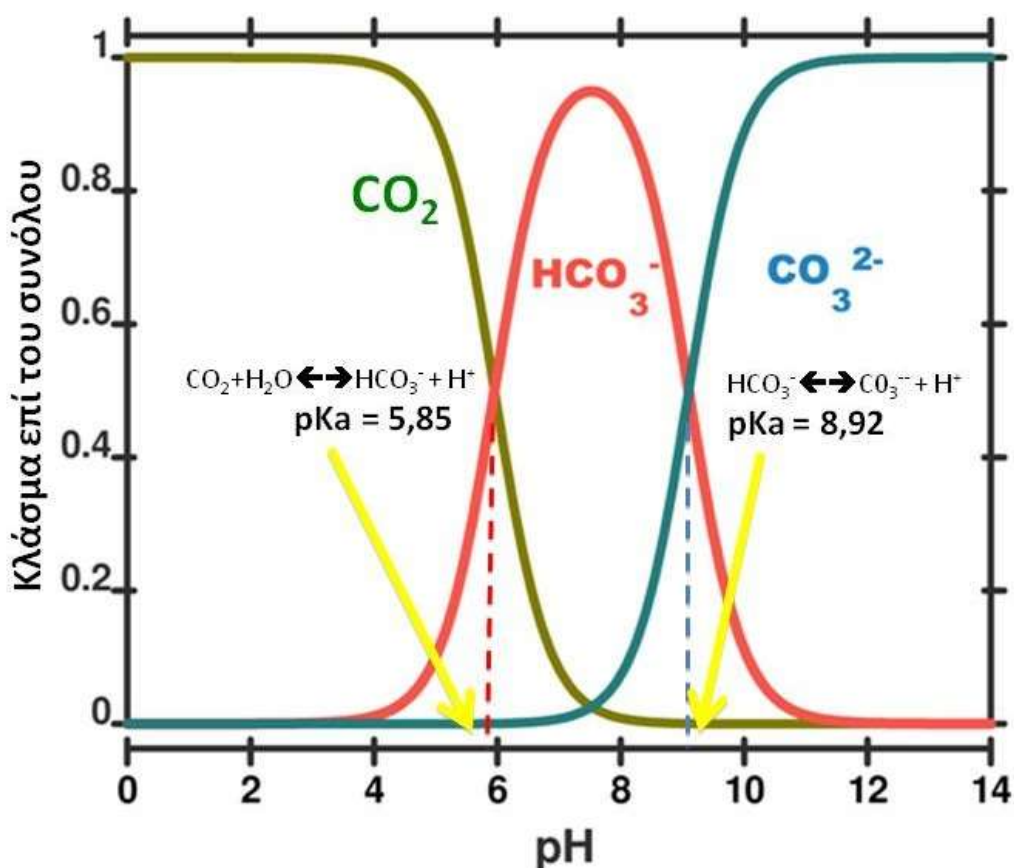
Σχήμα 2.38. Το σύστημα του διοξειδίου του άνθρακα συναρτησει του pH.
