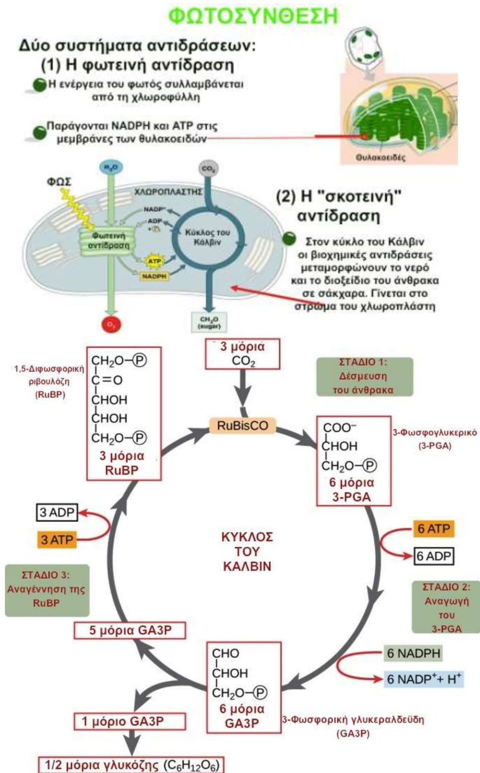
Σχήμα 12. Σχηματική συνοπτική απεικόνιση των φωτεινών και «σκοτεινών» αντιδράσεων της φωτοσύνθεσης (άνω σχήμα) και ο κύκλος του Κάλβιν (κάτω σχήμα).
