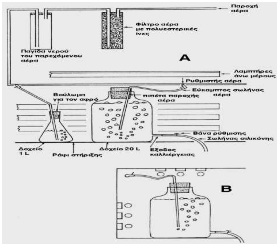
Σχήμα 17. Γενική σχεδιαγραμματική απεικόνιση της παροχής του αέρα και των φωτιστικών σωμάτων στα δοχεία καλλιέργειας φυτοπλαγκτού.
