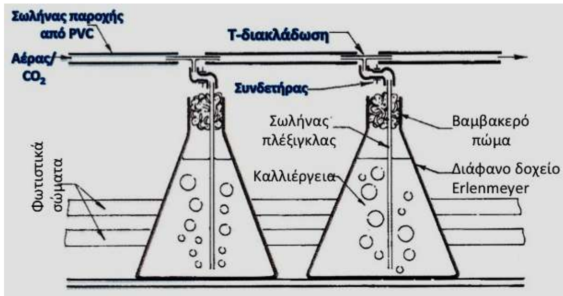
Σχήμα 15. Δοχεία καλλιέργειας φυτοπλαγκτού κυλινδροκωνικά τύπου Erlenmeyer με παροχή αέρα και λαμπτήρες.
