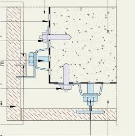
Τομή Υλικότητας
