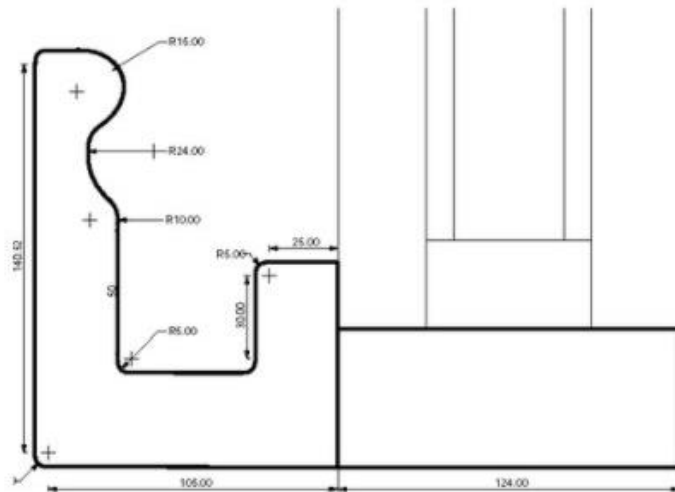
Door Handle Detail
