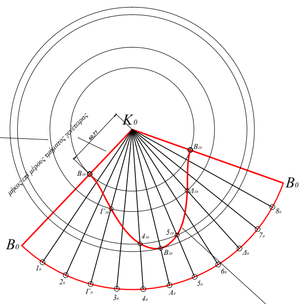
ΑΝΑΠΤΥΓΜΑ ΚΩΝΟΥ ΕΚ ΠΕΡΙΣΤΡΟΦΗΣ ΚΑΙ ΜΕΤΑΣΧΗΜΑΤΙΣΜΕΝΗ ΤΟΜΗΣ
