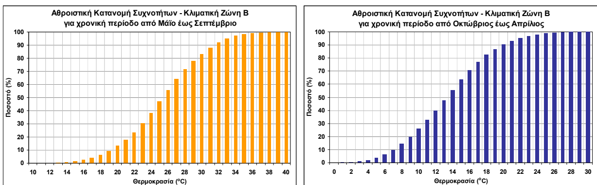
Σχήμα 2.2. Αθροιστική κατανομή συχνότητων θερμοκρασίας εξωτερικού αέρα για την Κλιματική Ζώνη Β.
