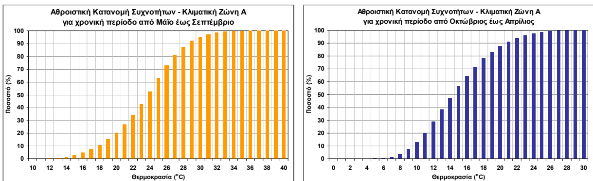
Σχήμα 2.1. Αθροιστική κατανομή συχνότητων θερμοκρασίας εξωτερικού αέρα για την Κλιματική Ζώνη Α.
