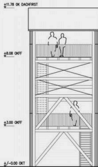
ANSICHT OST
