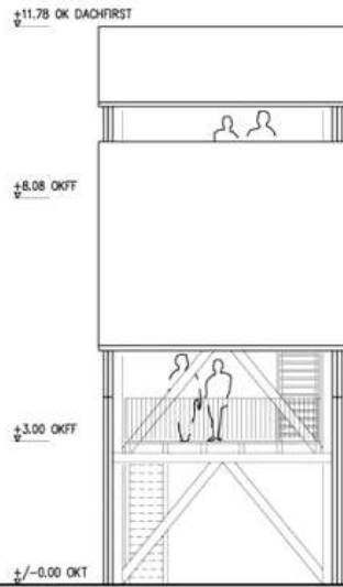
ANSICHT WEST
